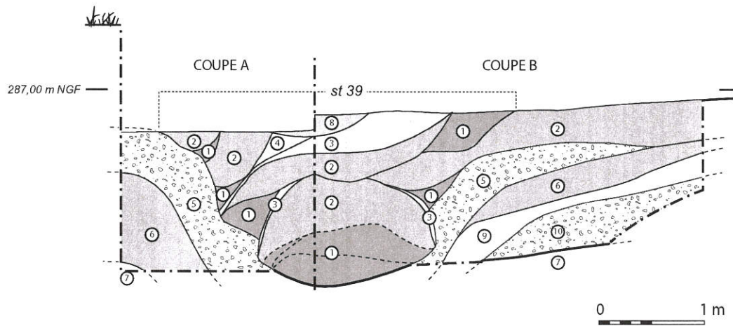
Fig. 27 : plan et coupe de st 39.
