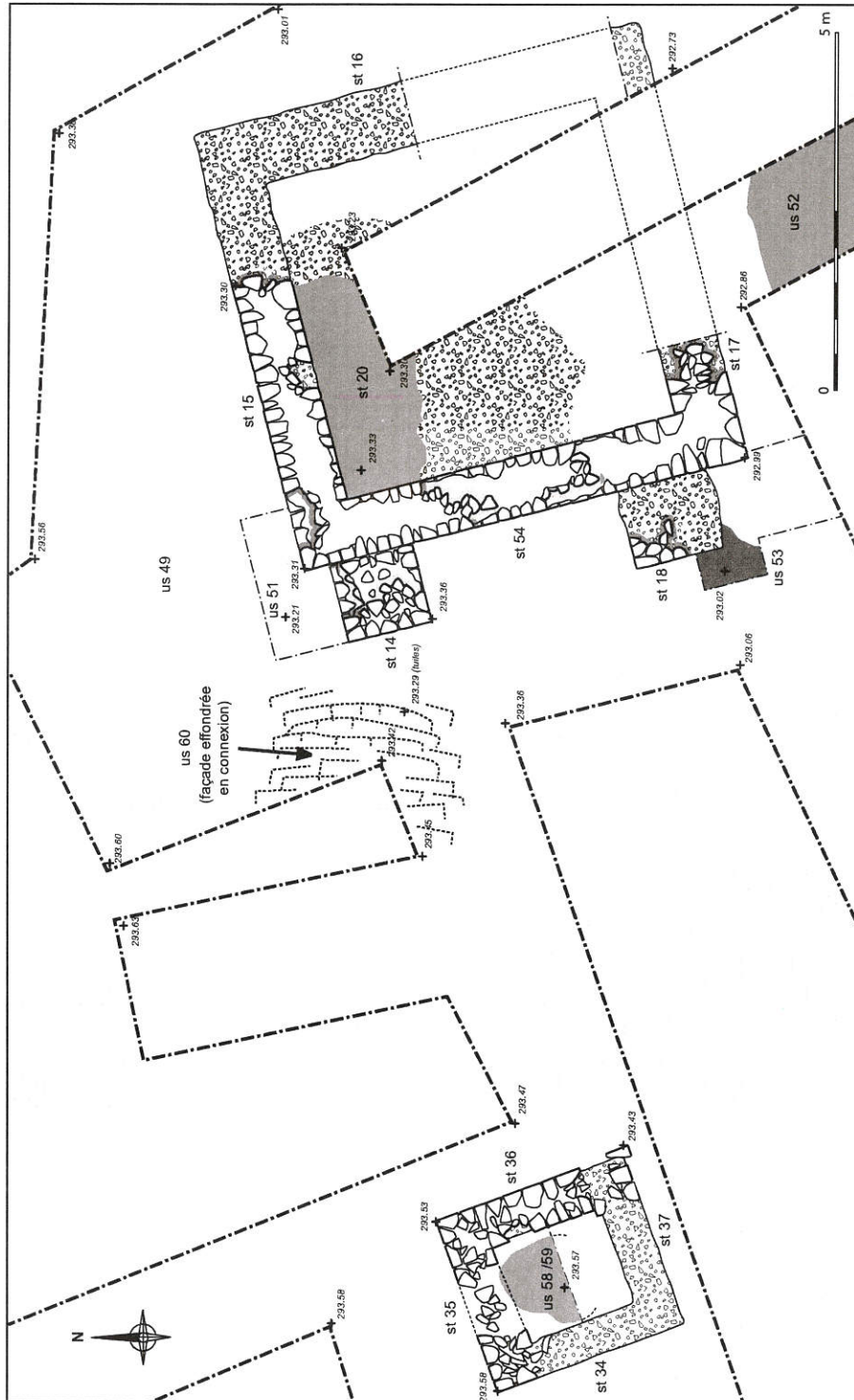
Fig. 5 : Plan du secteur des bâtiments 1 et 2.
