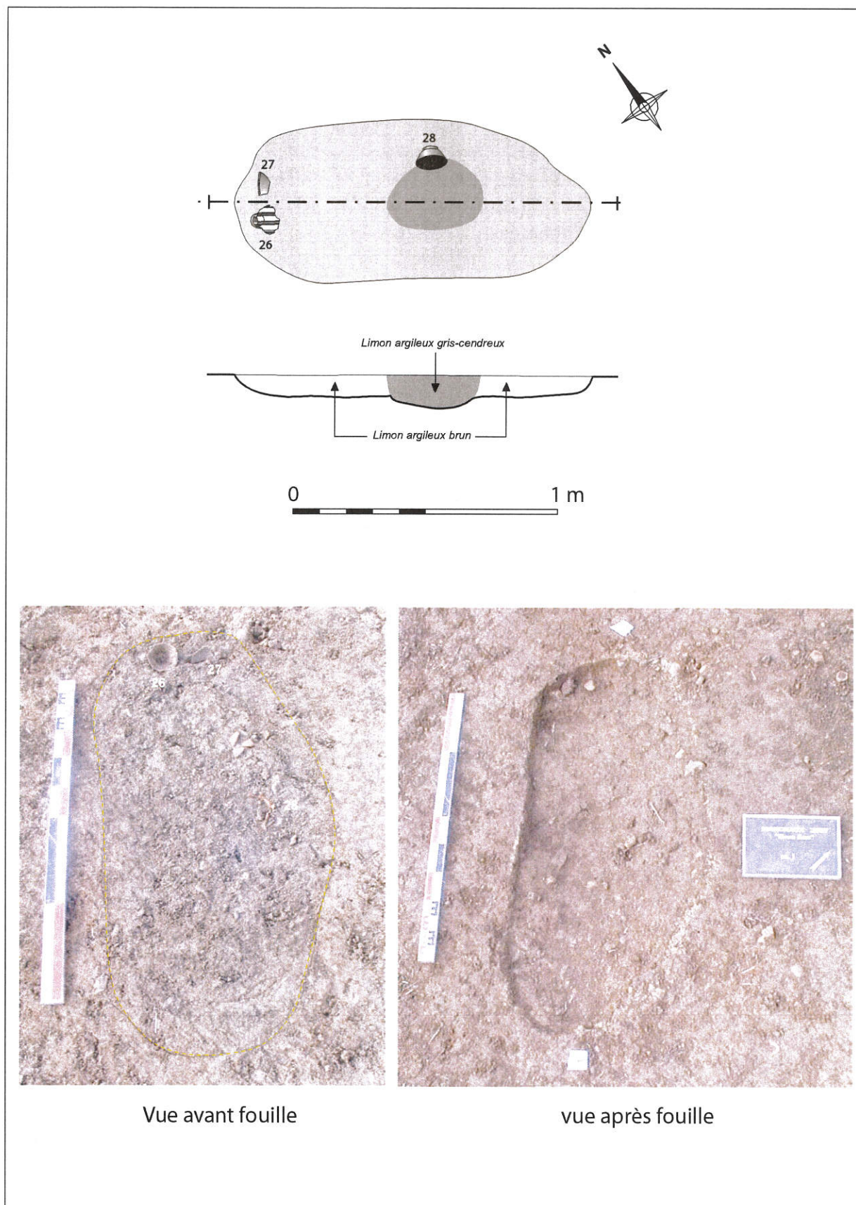
Fig. 22 : Plan, coupe et vues de la sépulture st 1.
