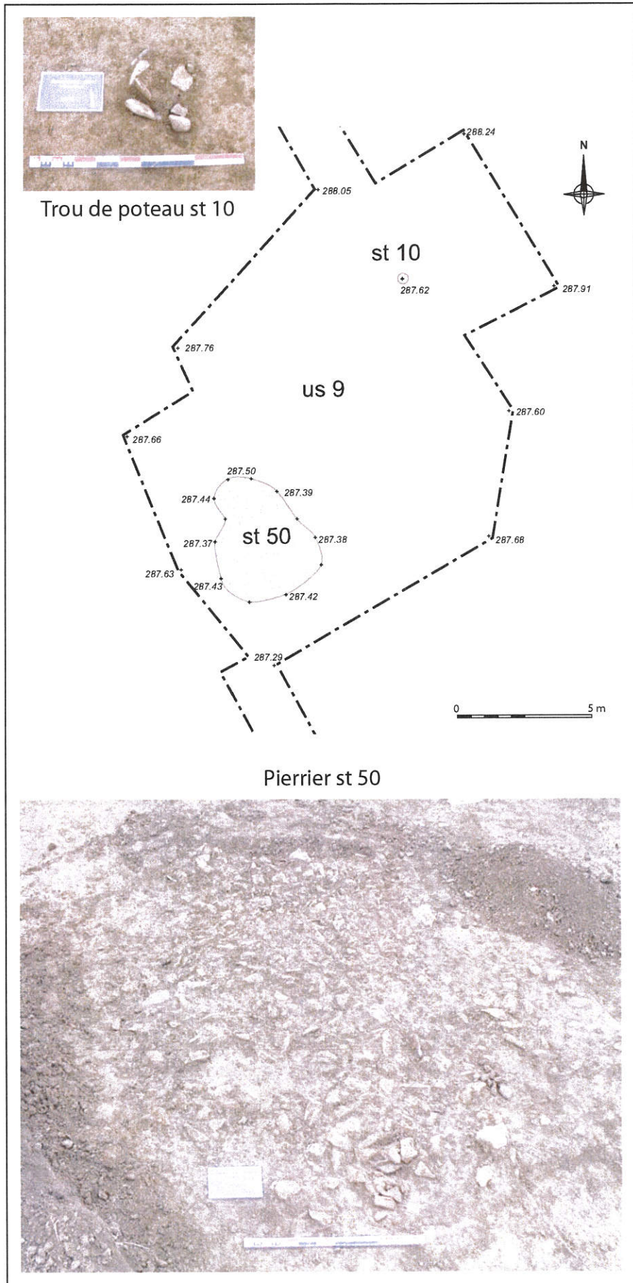
Fig. 24 : Plan et vues de la zone C.
