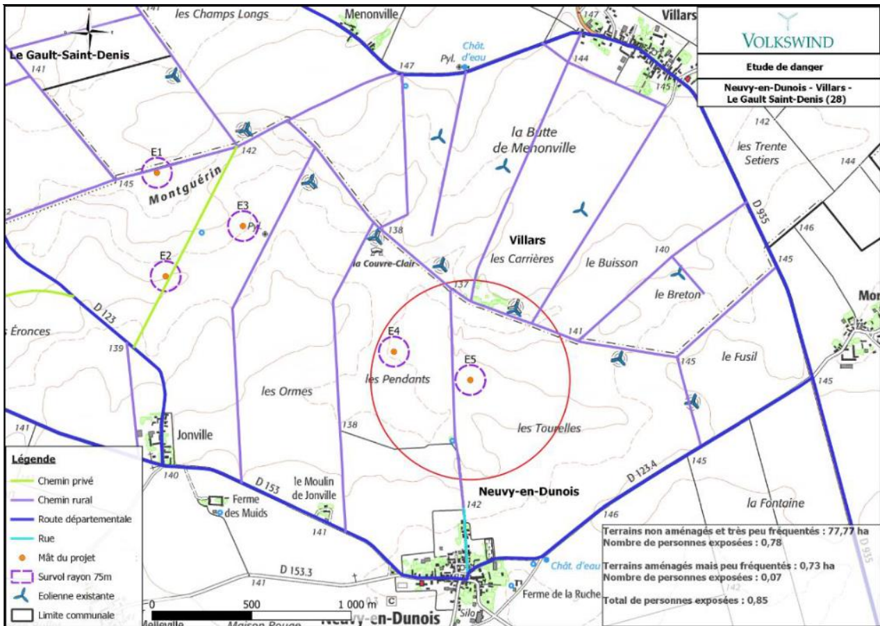
Carte 23 : Synthèse des cibles et du nombre de personnes exposées pour l'éolienne E5
