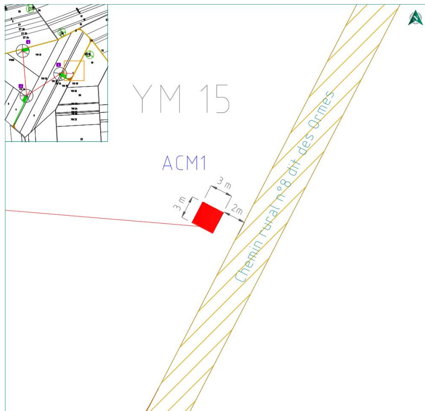
Carte 27 : Plan d'installation de l'armoire de coupure n°1
