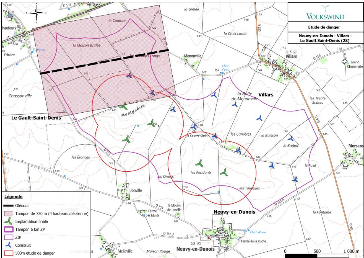
Carte 17 : Localisation de l'oléoduc dans la zone de projet
