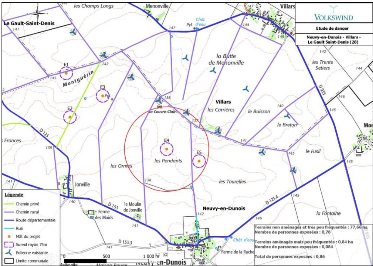
Carte 22 : Synthèse des cibles et du nombre de personnes exposées pour l'éolienne E4
