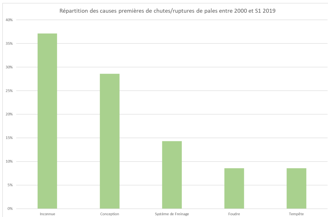
Figure 16 : Répartition des causes de chutes / ruptures de pales en France
