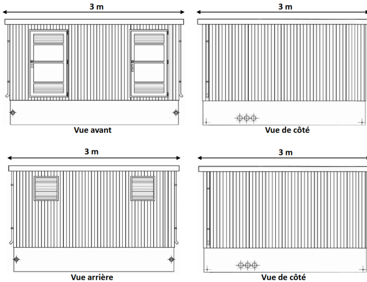
Figure 9 : Schéma d'une armoire de coupure (3 m x 3 m)
