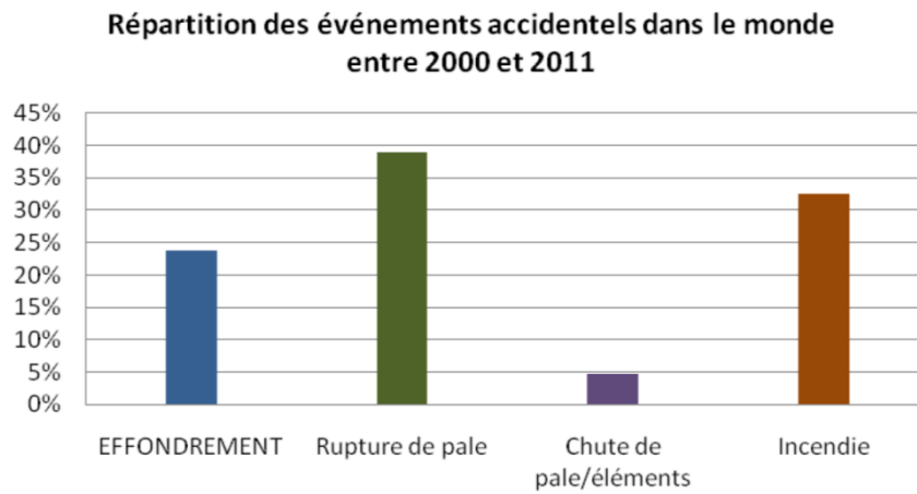
Figure 17 : Répartition des événements accidentels dans le monde
