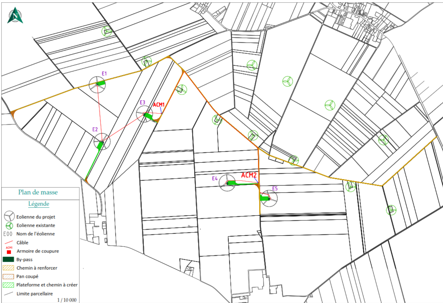
Carte 26 : Localisation des armoires de coupure et du réseau interne du parc éolien
