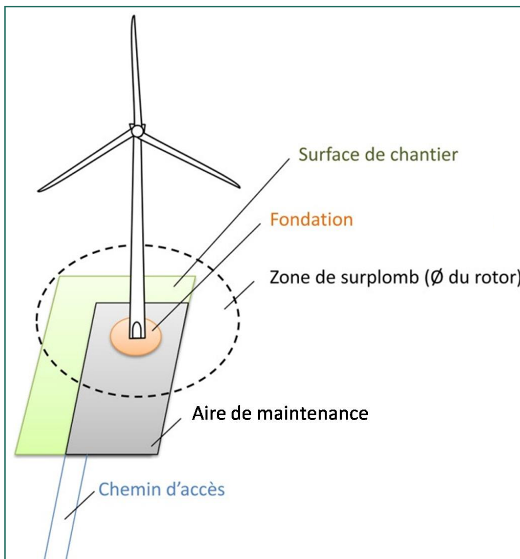
Figure 6 : Illustration des emprises au sol d'une éolienne (les dimensions sont données à titre d'illustration pour une éolienne d'environ 180m de hauteur)
