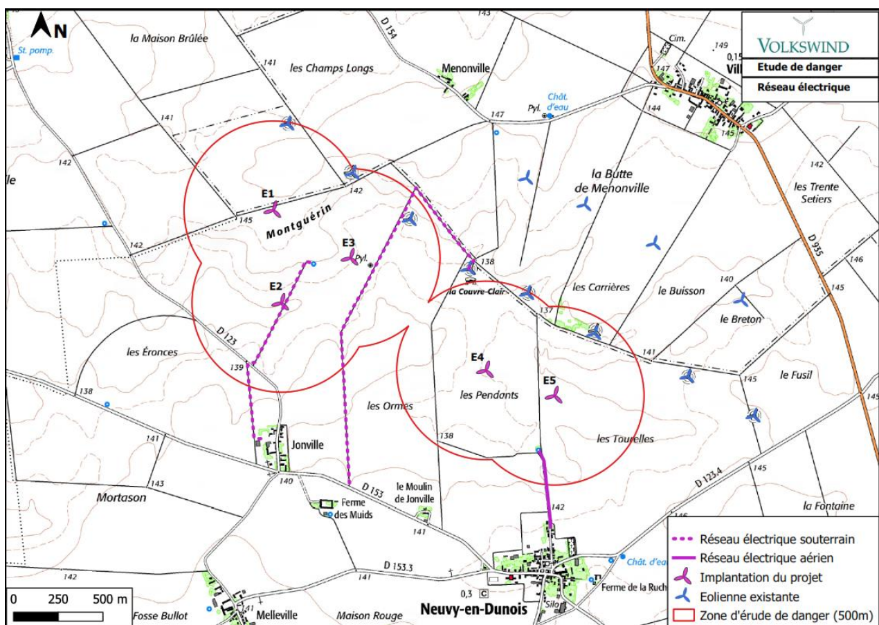
Carte 14 : Réseaux électriques
