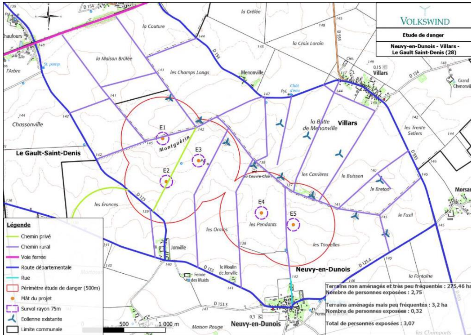
Carte 18 : Synthèse des cibles et du nombre de personnes exposées pour l'ensemble du parc
