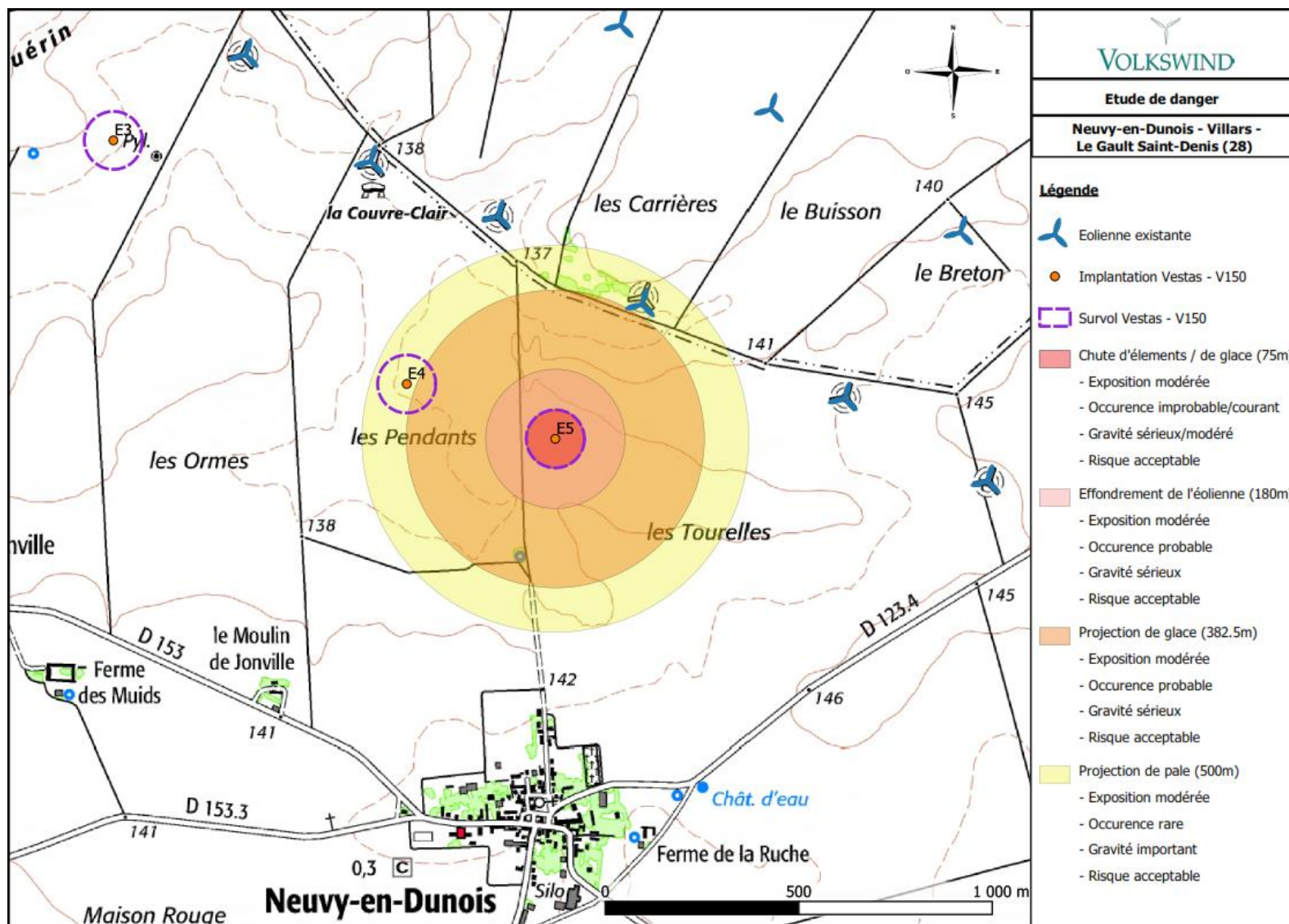
Carte 33 : Synthèse des risques pour l'éolienne E5
