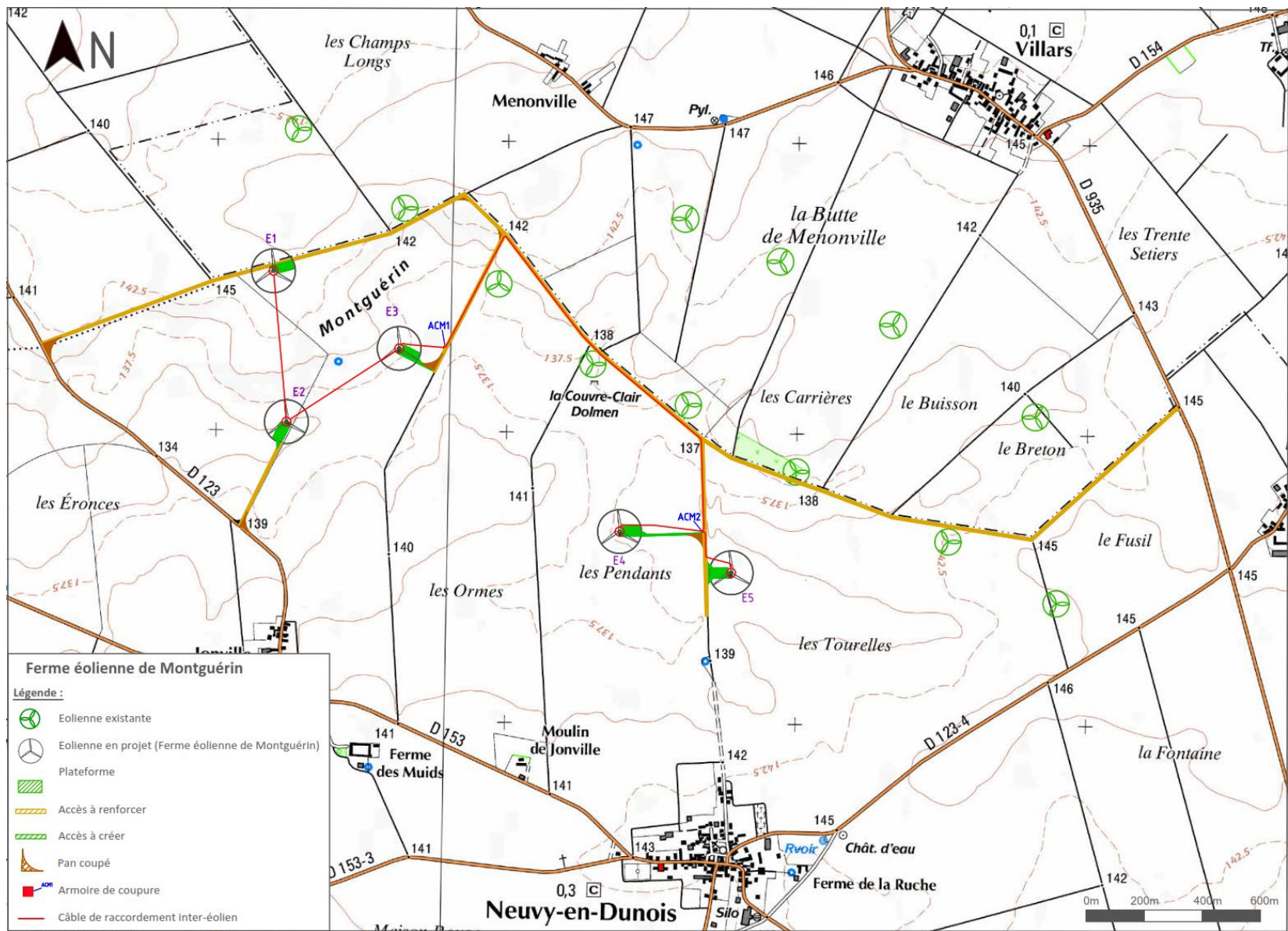
Carte 24 : Implantation du parc éolien
