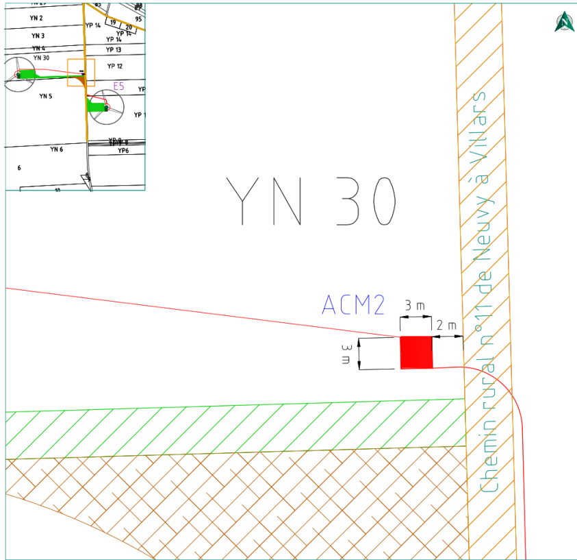
Carte 28 : Plan d'installation de l'armoire de coupure n°2
