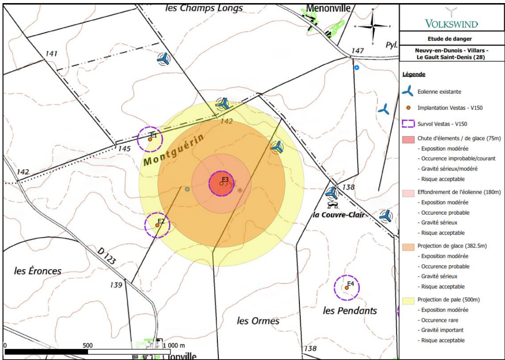
Carte 31 : Synthèse des risques pour l'éolienne E3
