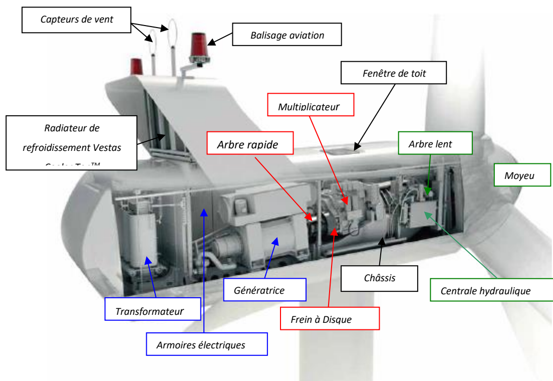
Figure 3 : Schéma technique de la nacelle Vestas V150
