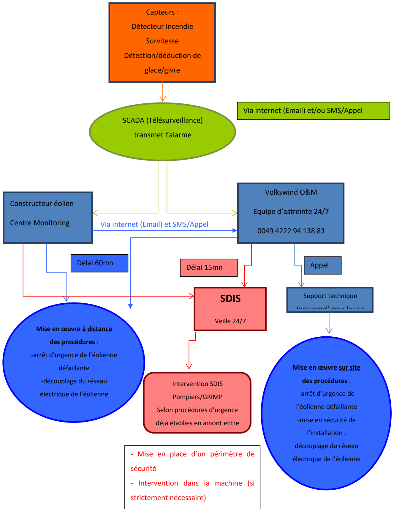
Figure 12 : Procédure en cas d'incident
