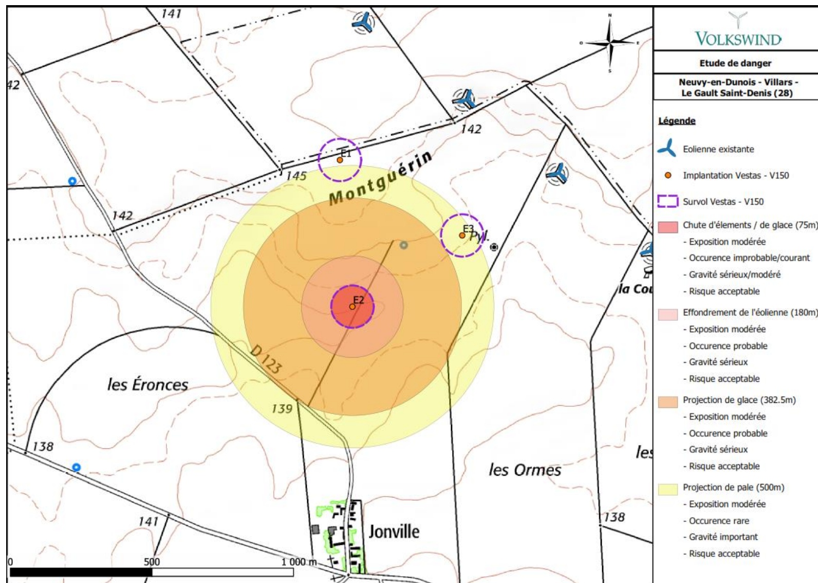
Carte 30 : Synthèse des risques pour l'éolienne E2
