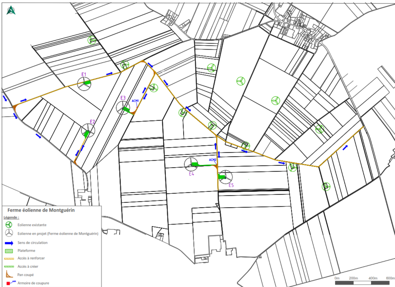
Carte 25 : Voies d'accès aux éoliennes - Plan cadastral (voie d'accès)
