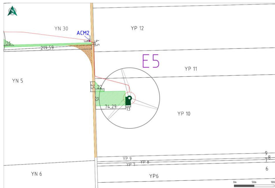
Figure 7 : Aires de montage et d'entretien des éoliennes
