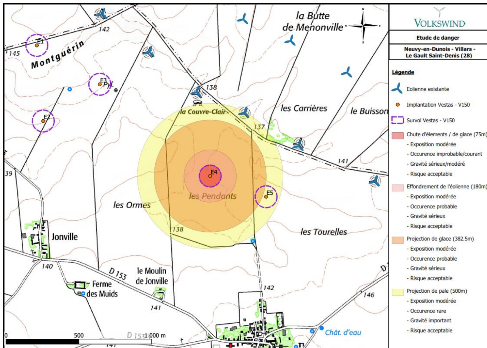
Carte 32 : Synthèse des risques pour l'éolienne E4
