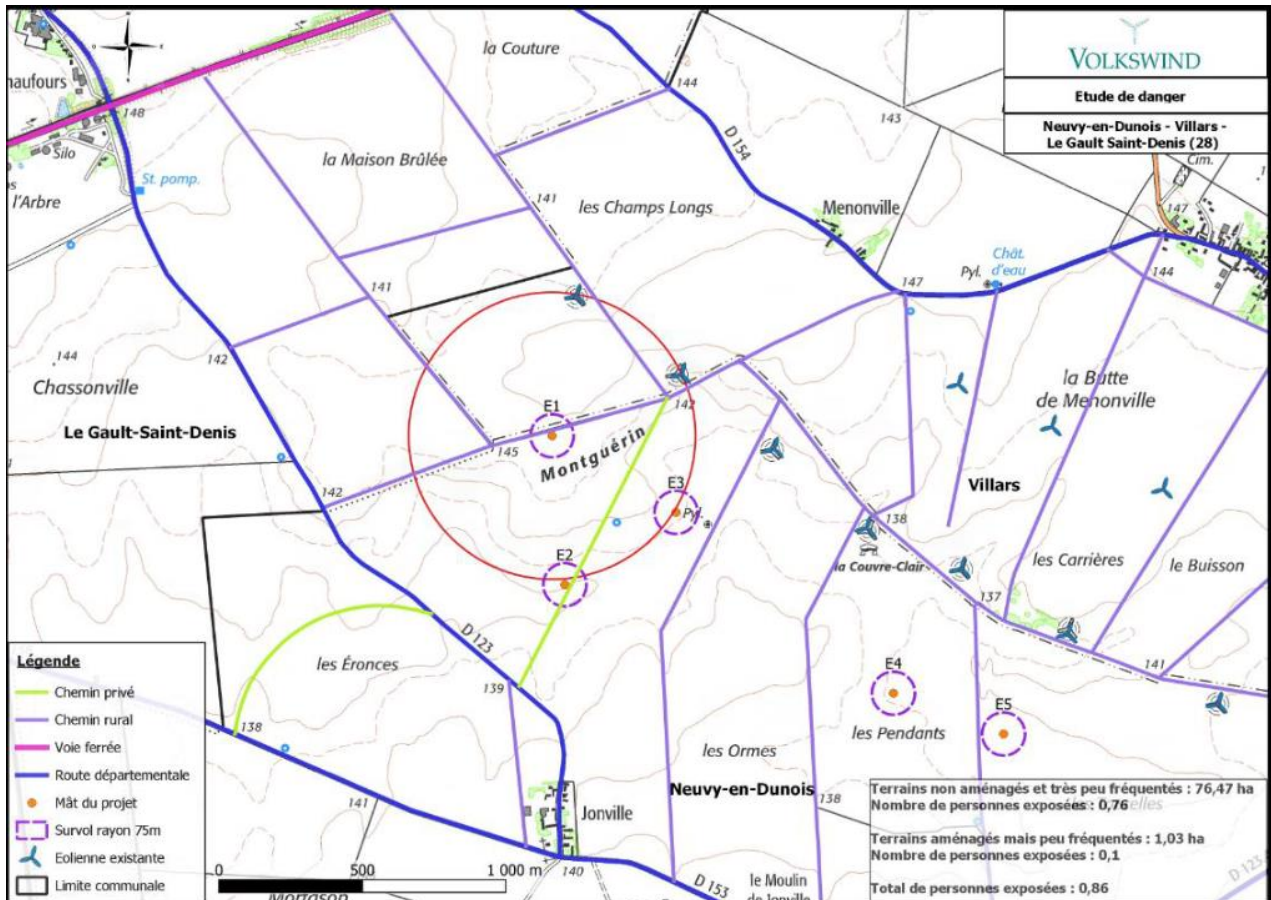
Carte 19 : Synthèse des cibles et du nombre de personnes exposées pour l'éolienne E1
