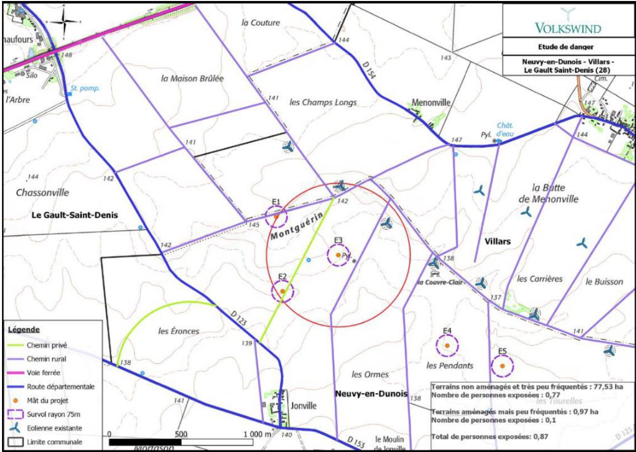
Carte 21 : Synthèse des cibles et du nombre de personnes exposées pour l'éolienne E3
