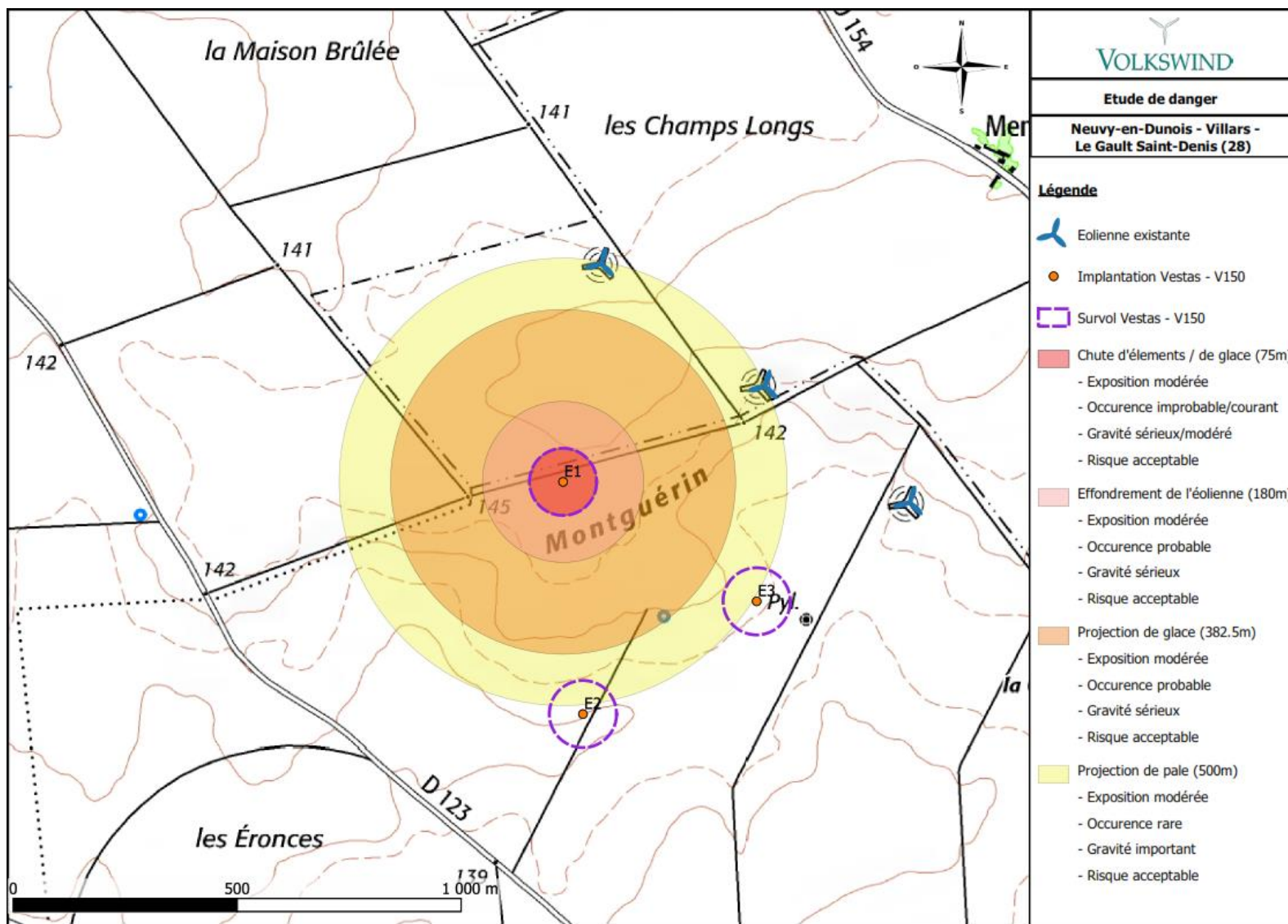
Carte 29 : Synthèse des risques pour l'éolienne E1
