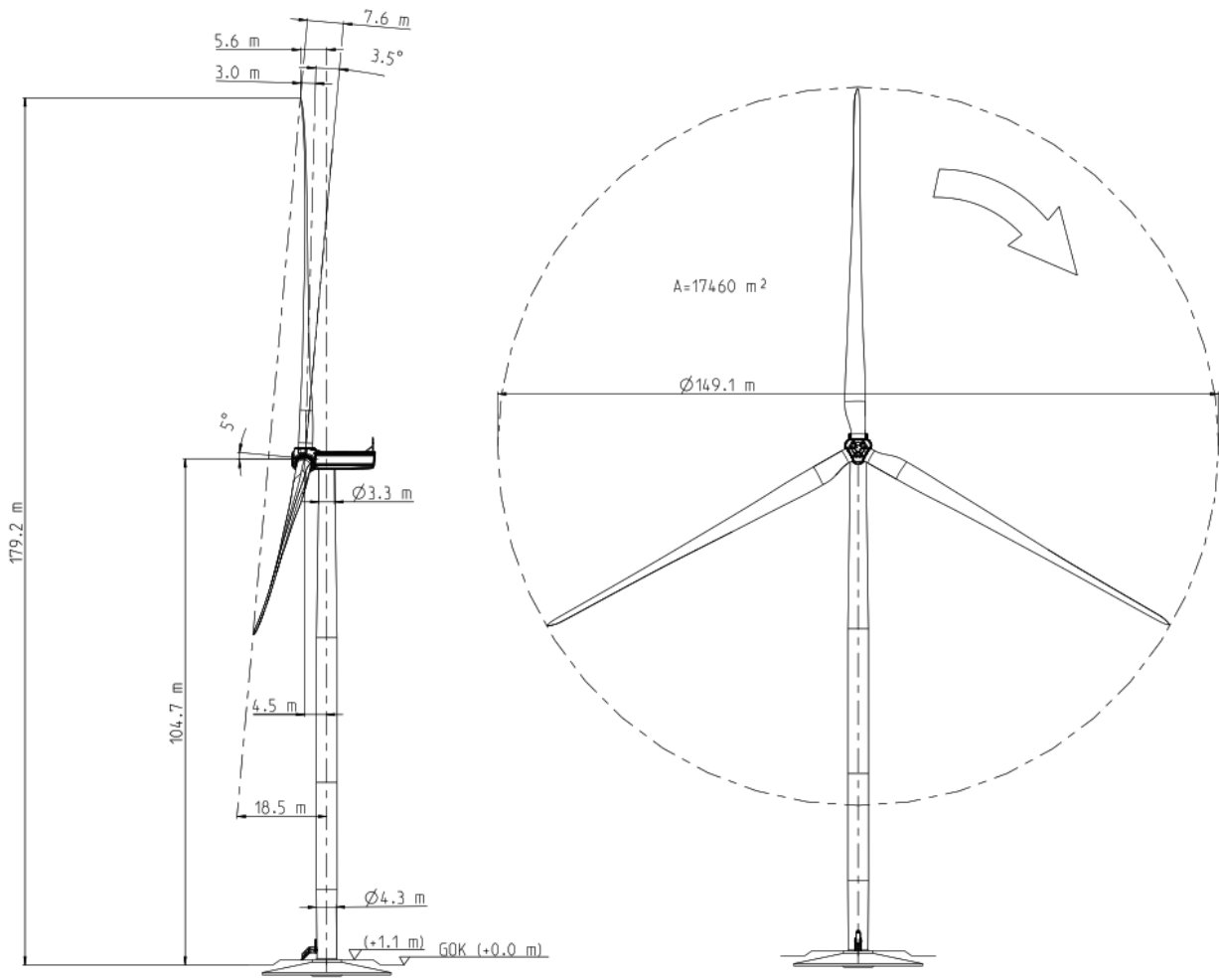
Figure 5 : Dessin d'élévation de l'éolienne Nordex N149- 4,5 MW
