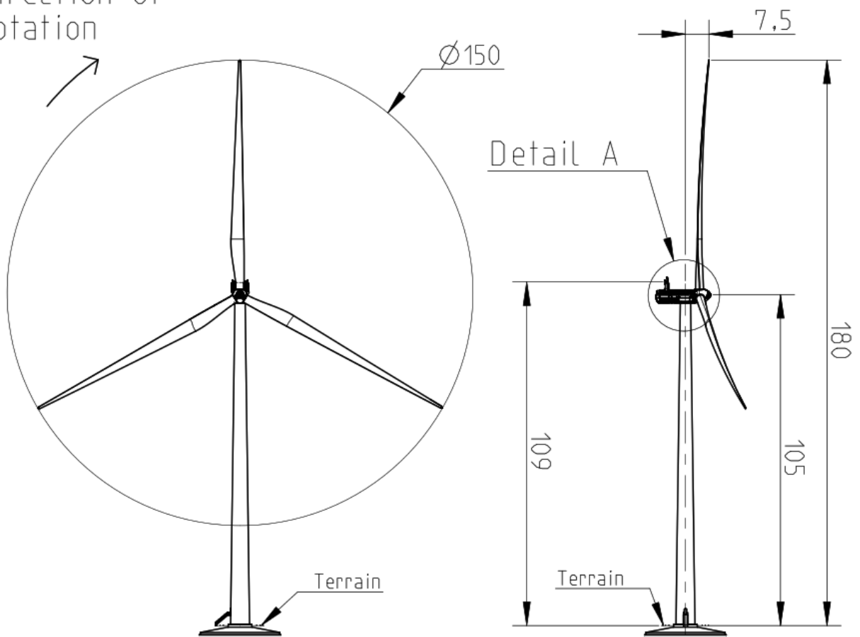
Figure 4 : Dessin d'élevation de l'éolienne Vestas V150- 4,2 MW
