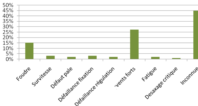
Figure 19 : Répartition des causes premières de rupture de pale
