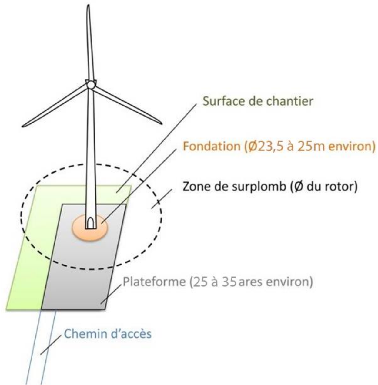
Figure 6 : Schéma de l'emprise au sol d'une éolienne (Source : Vestas)
