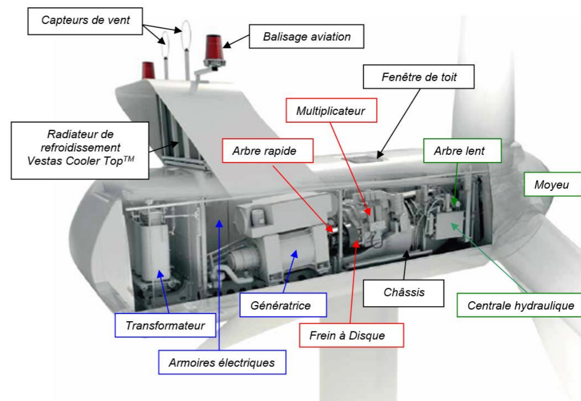
Figure 7 : Exemple de schéma illustrant les composants de la nacelle (Source : Vestas)
