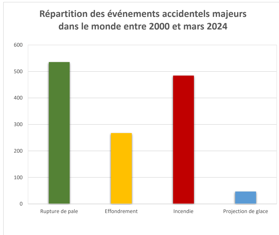
Figure 25 : Répartition des événements accidentels majeurs dans le monde entre 2000 et mars 2024
