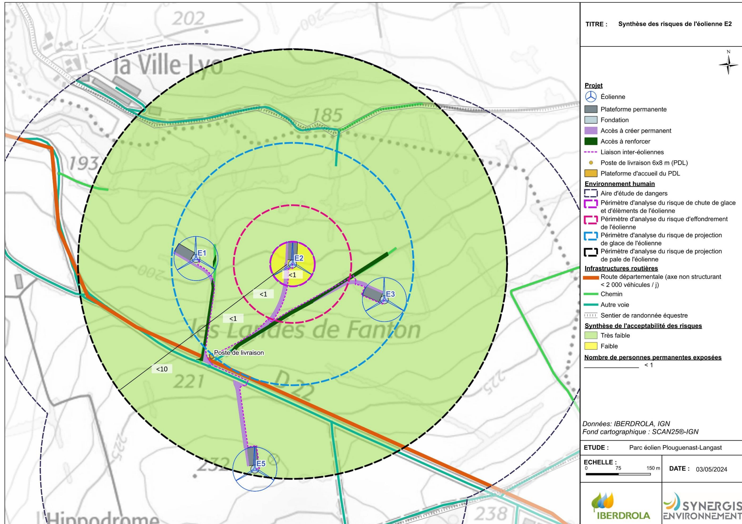
Figure 31 : Synthèse des risques de l'éolienne E2
