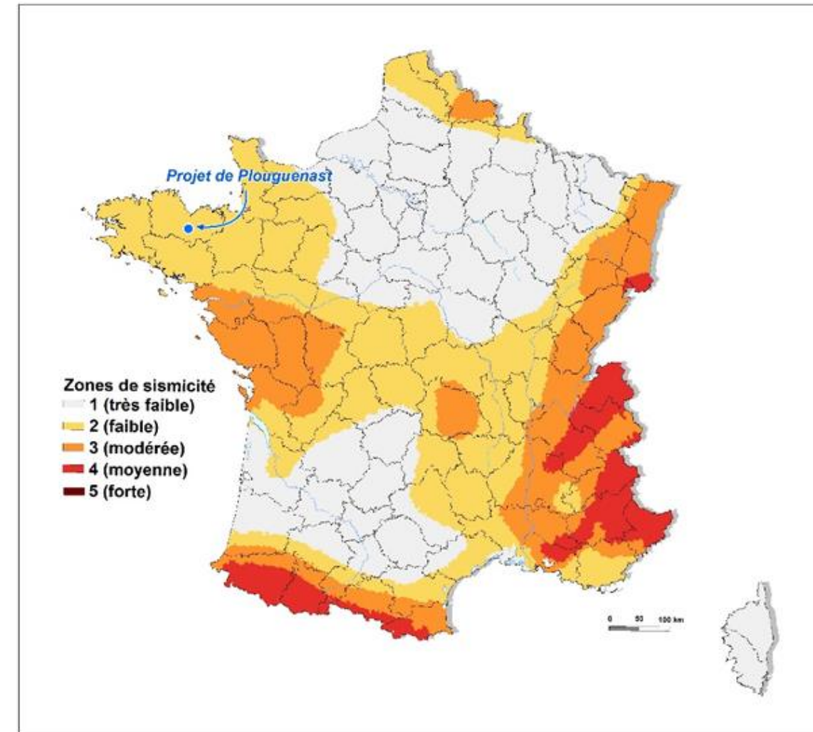
Figure 11 : Zonage sismique de la France (Source : BRGM)
