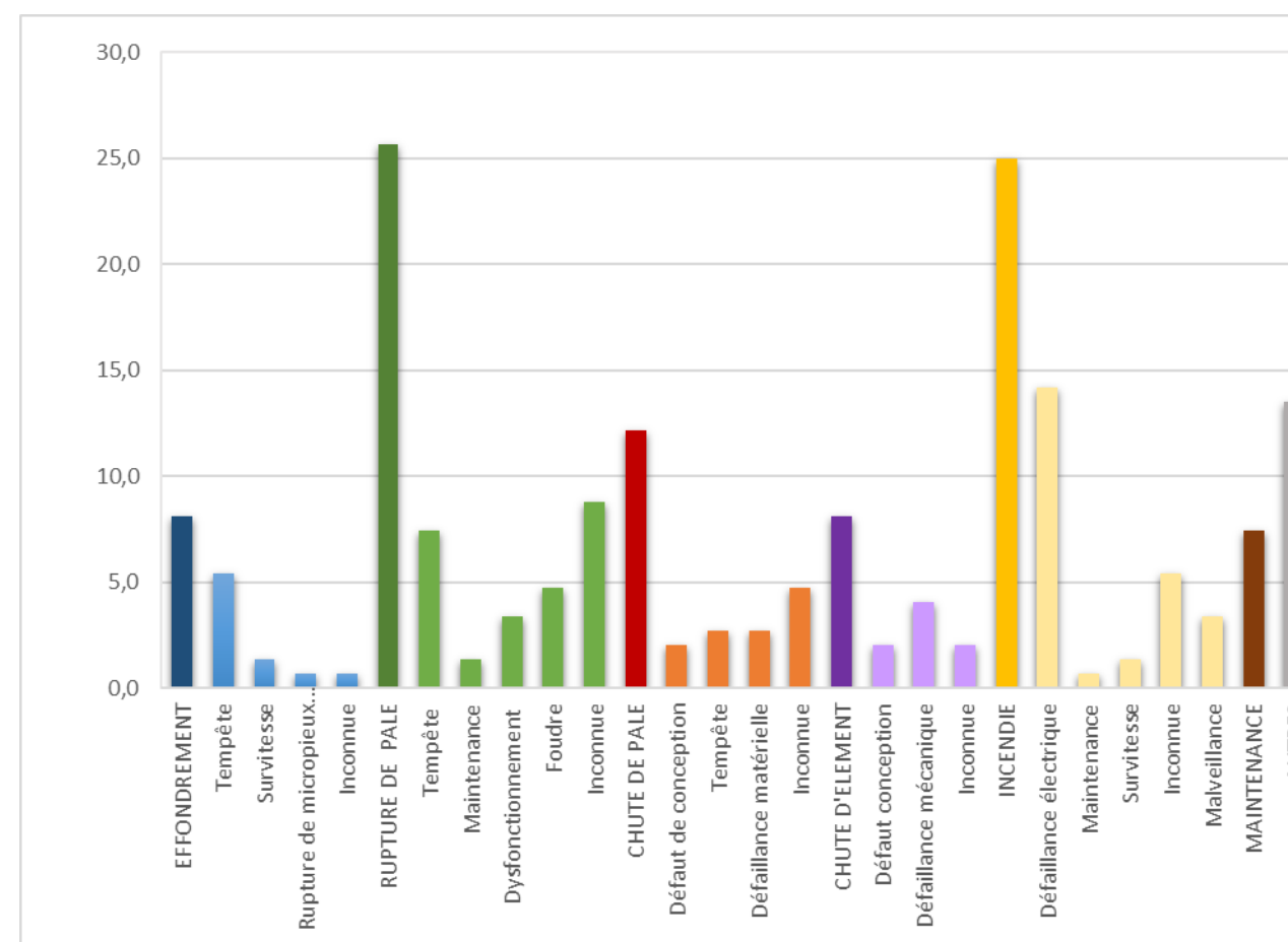
Figure 24 : Répartition des événements accidentels et de leurs causes premières sur le parc d'aérogénérateurs français entre 2000 et mars 2024
