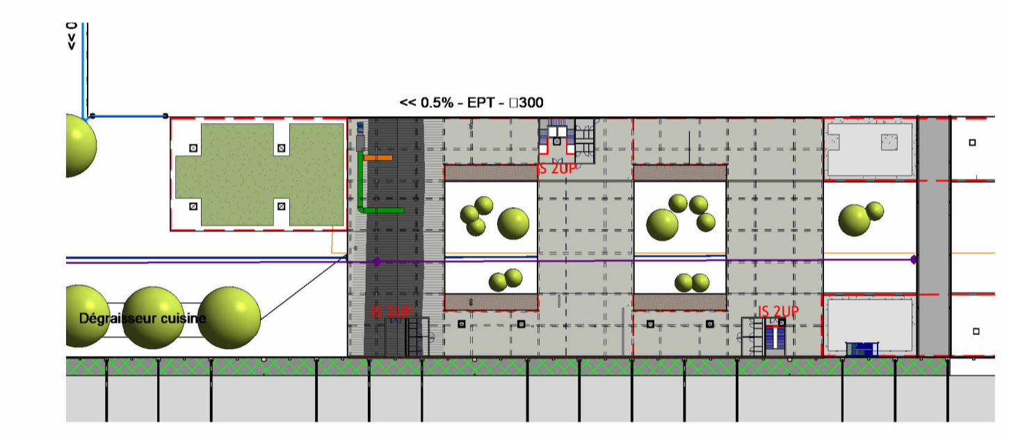
Niveau 01 - Bureaux Ech: 1:1000
