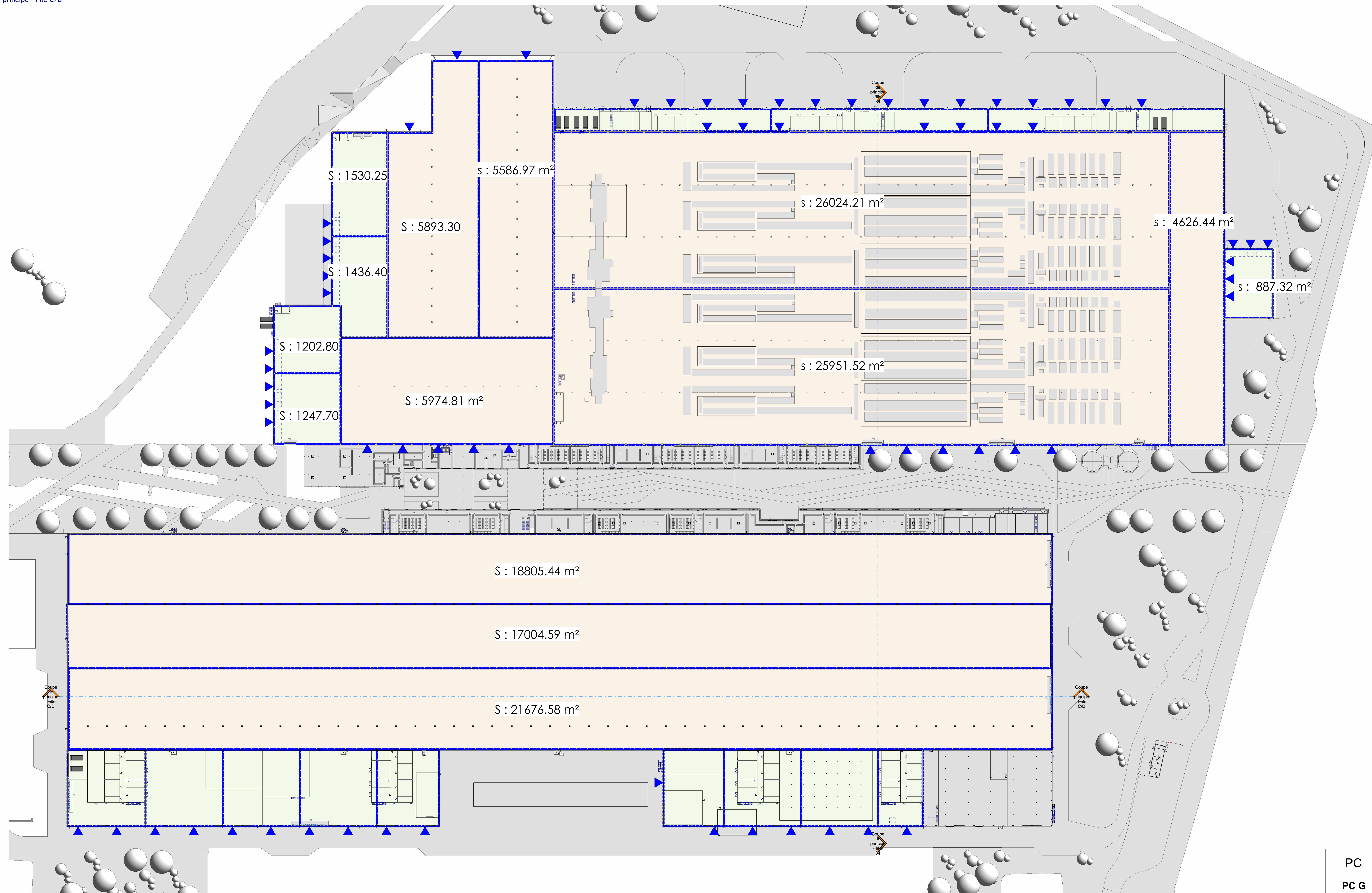
3 Niveau 0 - Sans Canton - Dépendante 1
