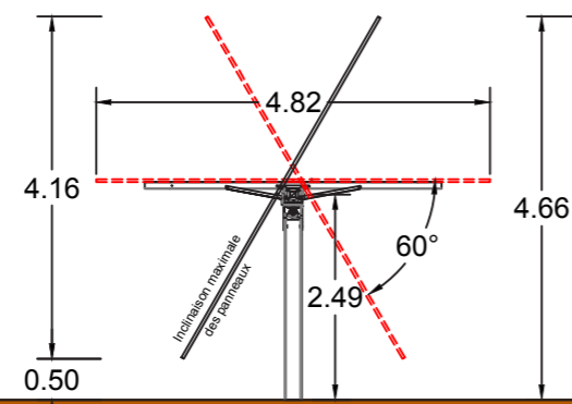
Vue latérale
