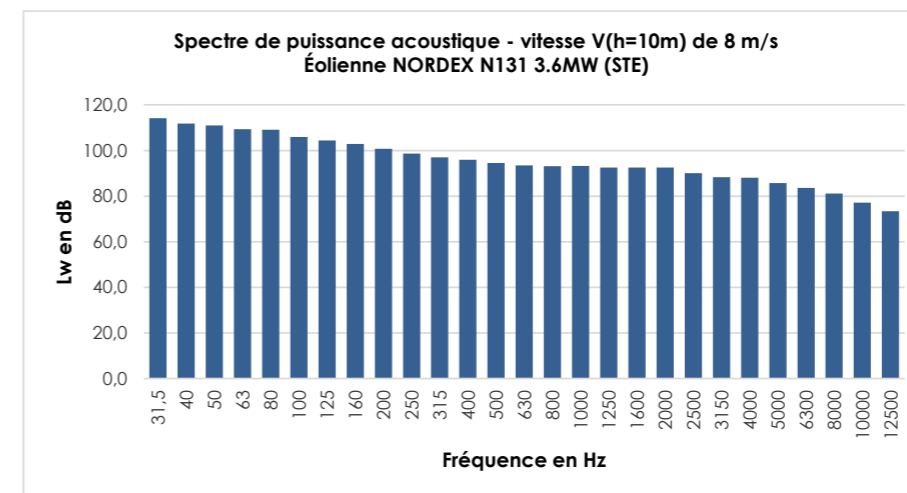
Figure 9. Graphique des niveaux de puissance acoustique d'une Nordex N131 3.6MW STE par bande de tiers d'octave à la vitesse de 8 m/s
