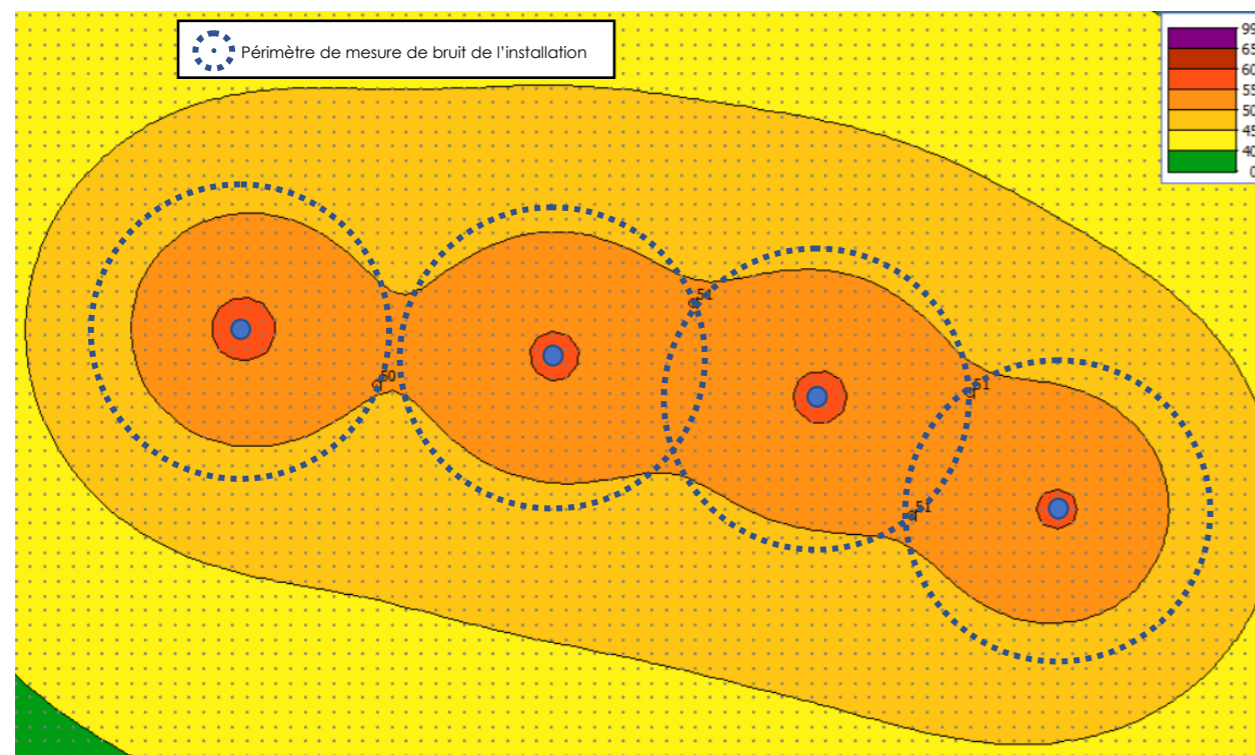
Figure 8. Cartographie sonore – Nordex N131 3.6MW STE
