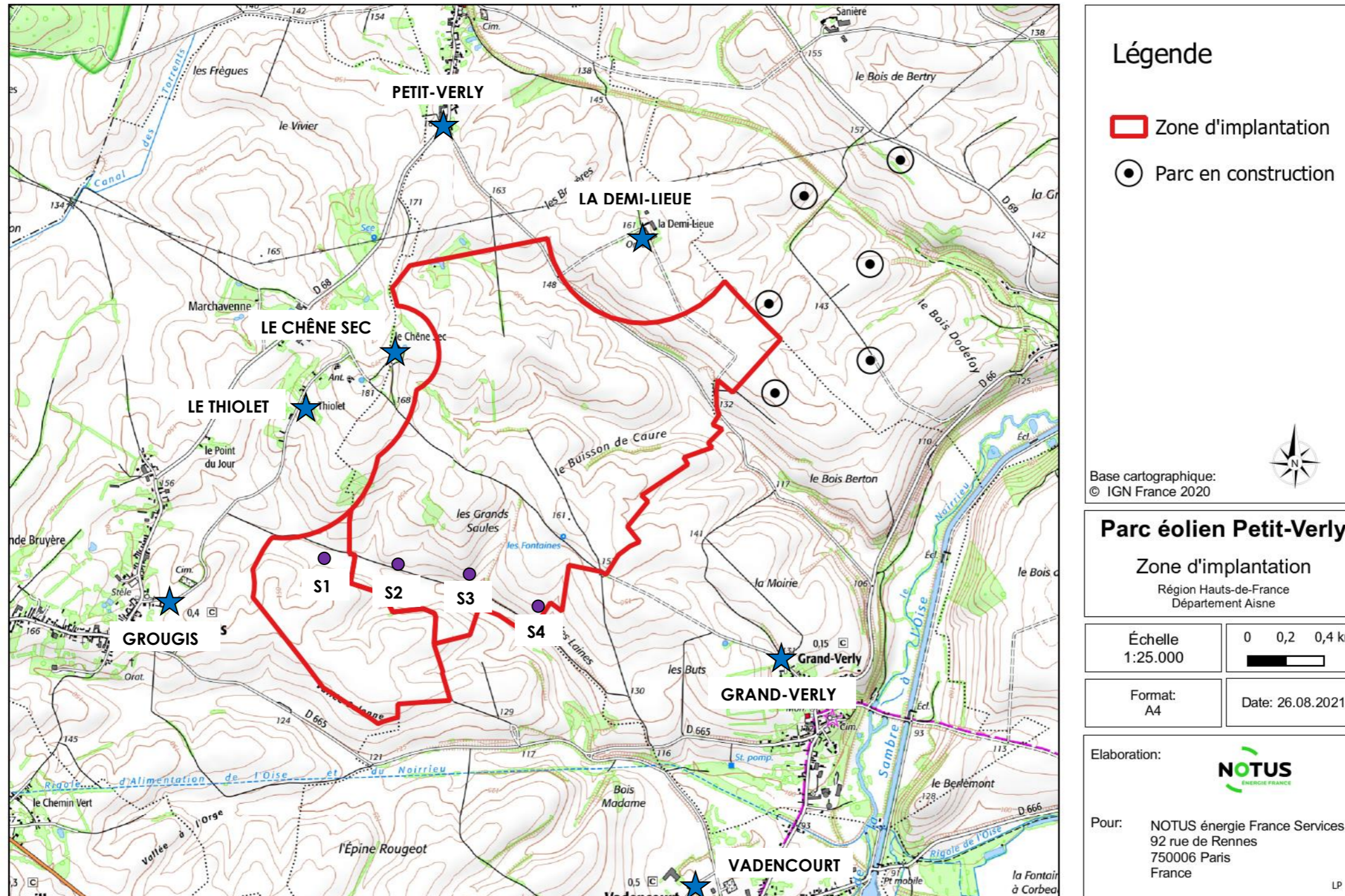
Figure 5. Implantation des points de contrôle et des éoliennes
