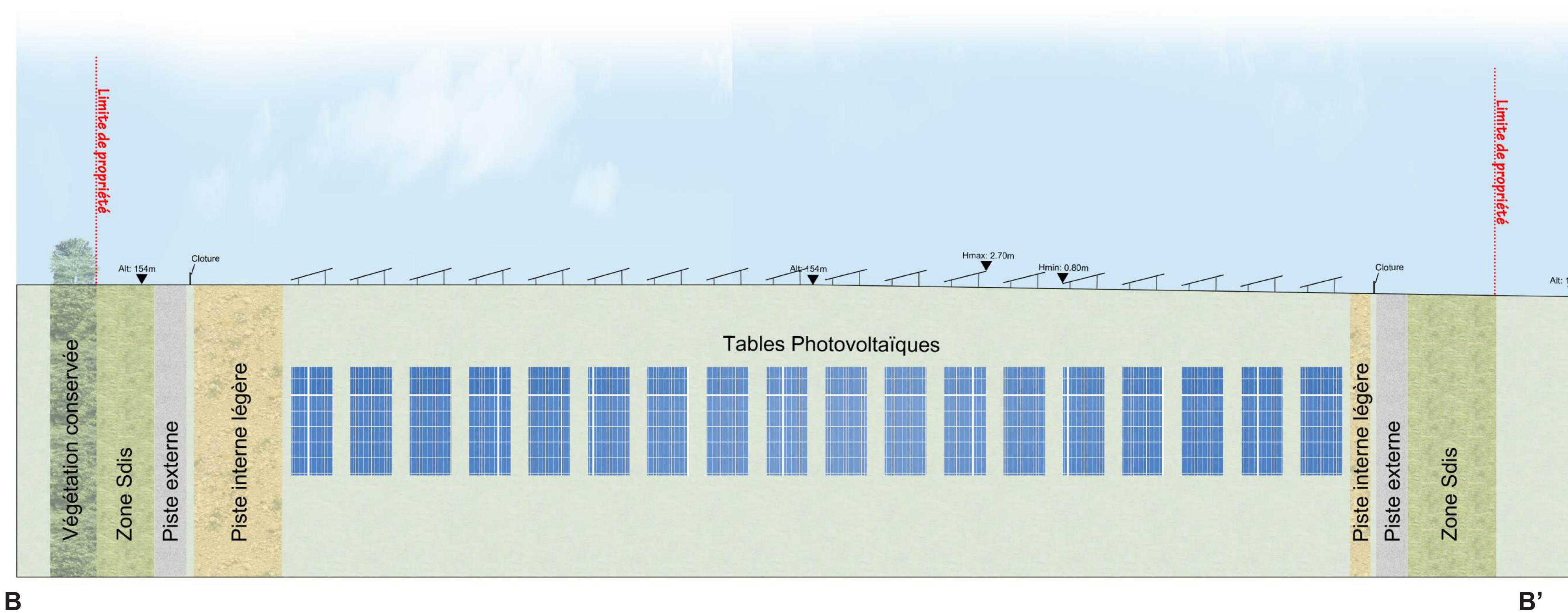
COUPE BB' : SUD / NORD DES PANNEAUX PHOTOVOLTAIQUES - échelle 1/500e
