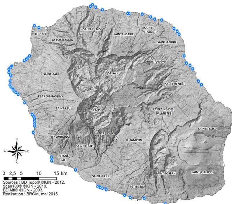
Figure 28 - Sites sensibles à l'action des houles (Chateauminois, 2015)
