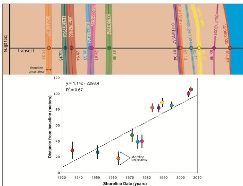
Figure 32 - Principe de la régression linéaire pondérée pour le calcul par DSAS de l'évolution du trait de côte (Himmelstoss, 2009)
