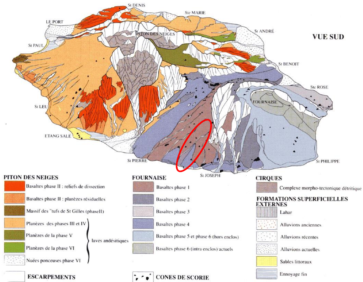
Figure 3 - Perspective morpho-géologique schématisée de La Réunion avec localisation de la commune de Petite-Île en rouge (modifié, Raunet, 1991)
