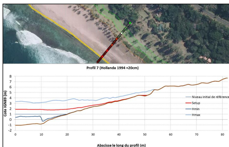
Figure 44 - Profils de plage, setup, Hmin et Hmax avec simulation du cyclone Hollanda + 20 cm profil 7 Petite-île
