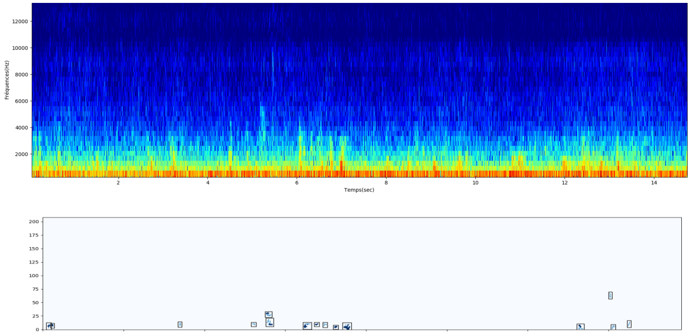
Figure 97. Représentation de 15 secondes de signal (10_08_18_bruit_bateau_voie.wav) contenant du bruit de bateau mais également la voix du guide sur ce bateau, en haut : signal brut, en bas, résultats du détecteur, qui a détectés des bruits anthropiques (bleu clair sur la voie 1 et bleu foncé sur la voie 2). Enregistrement disponible : http://sabiiod.univ-tln.fr/scandola_2018/10_08_18_bruit_bateau_voie.wav
