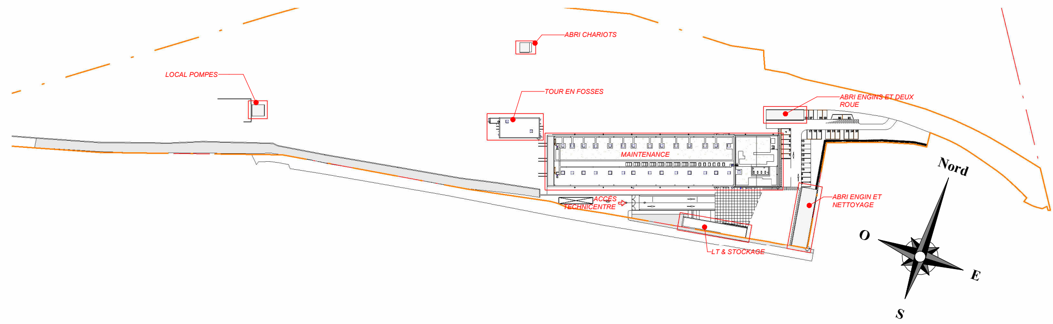
Plan de repérage 1 : 2000
