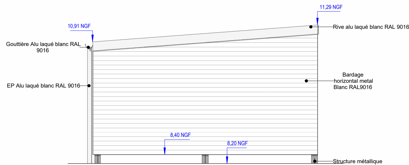
Elévation Sud abri chariots 1 : 50
