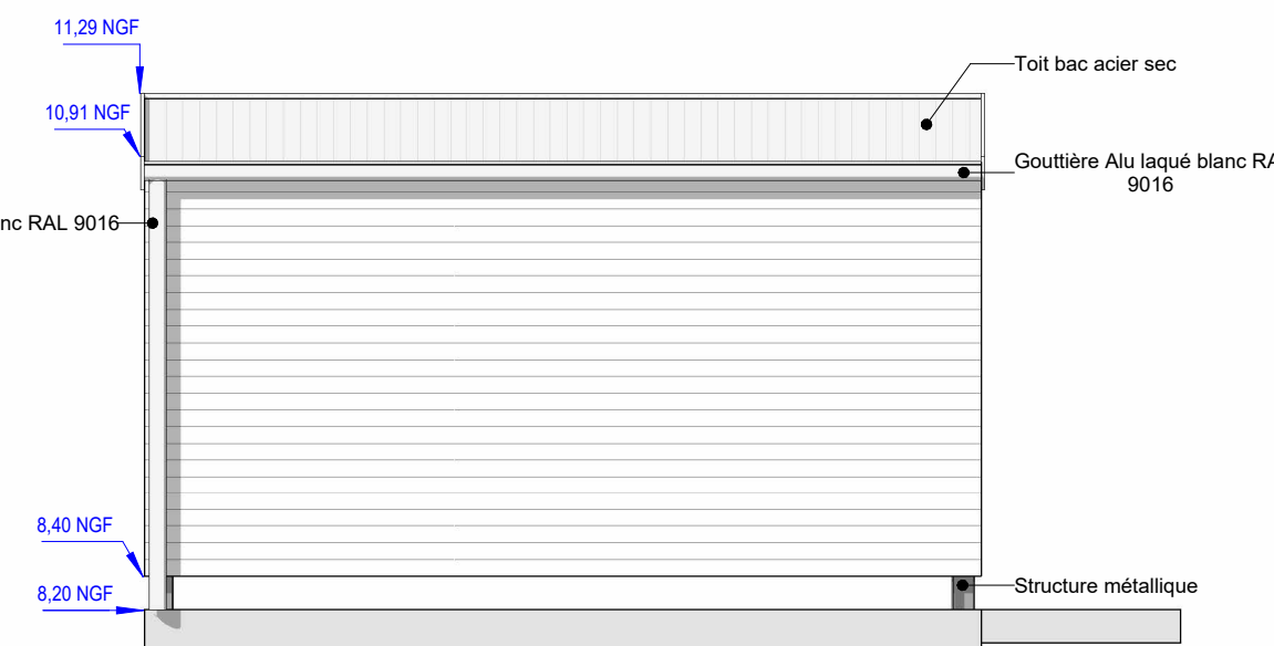
Elévation Ouest abri chariots 1 : 50
