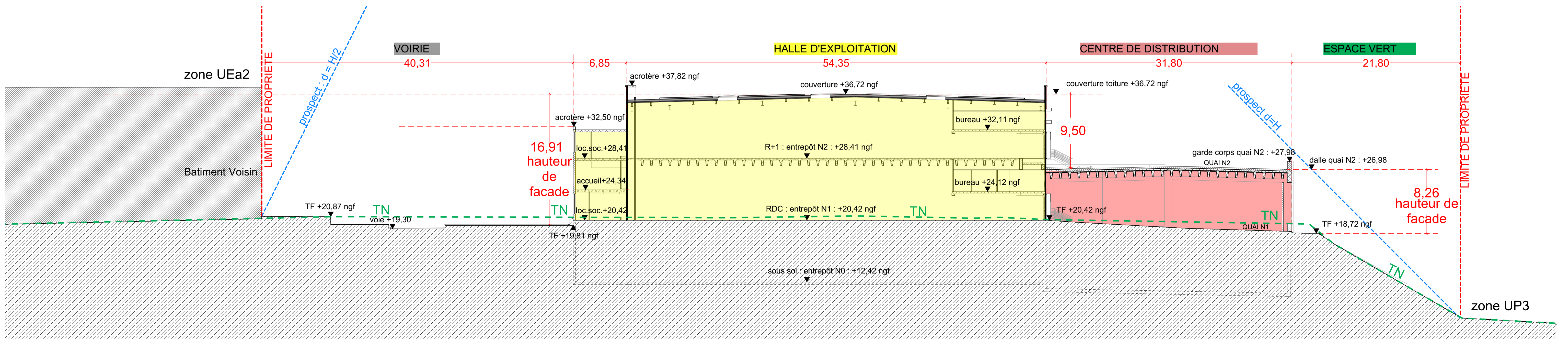
Coupe PC 3.3 - 1/250
