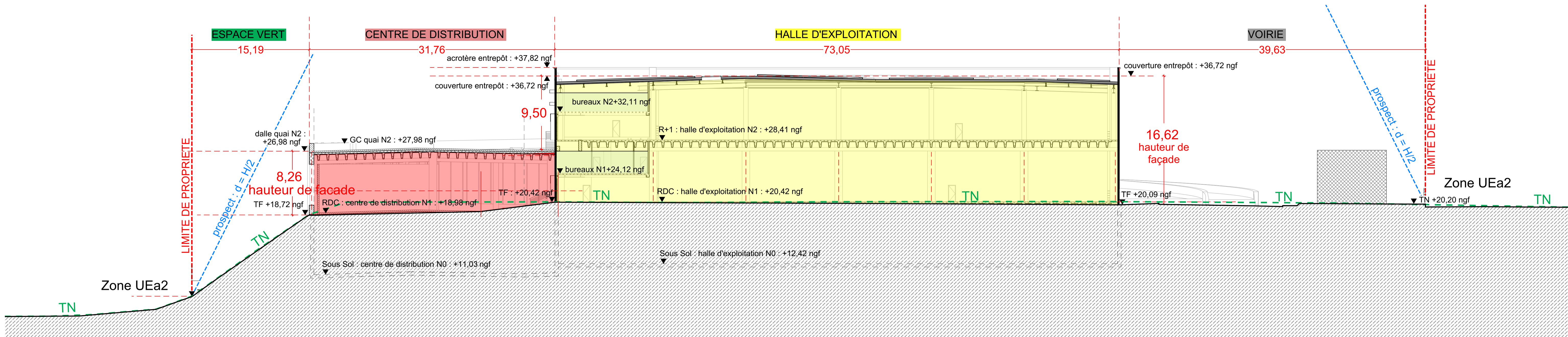
Coupe PC 3.1 - 1/250
