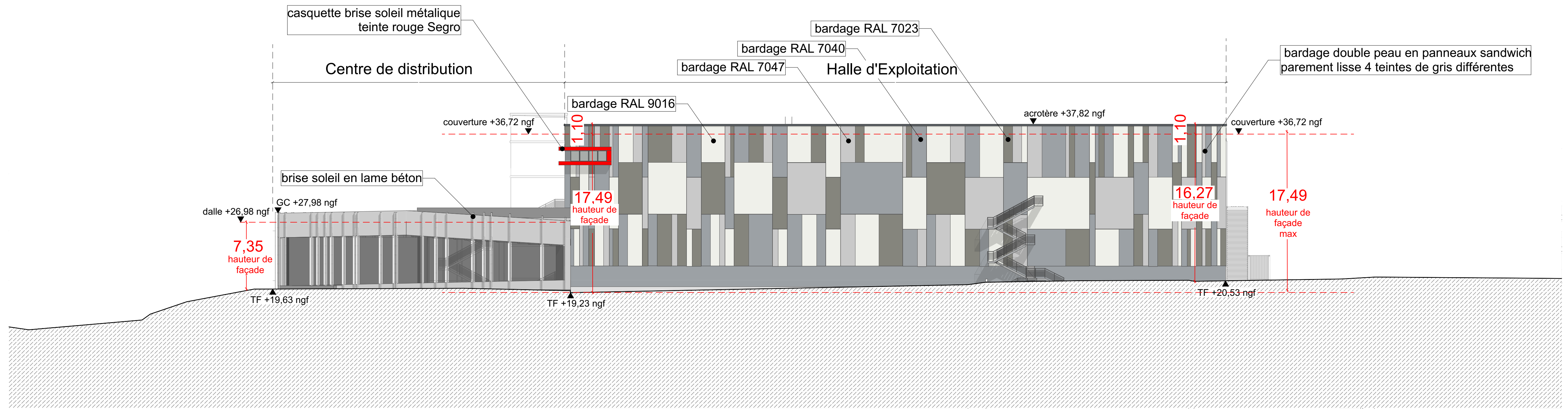
Facade Est - 1/250
