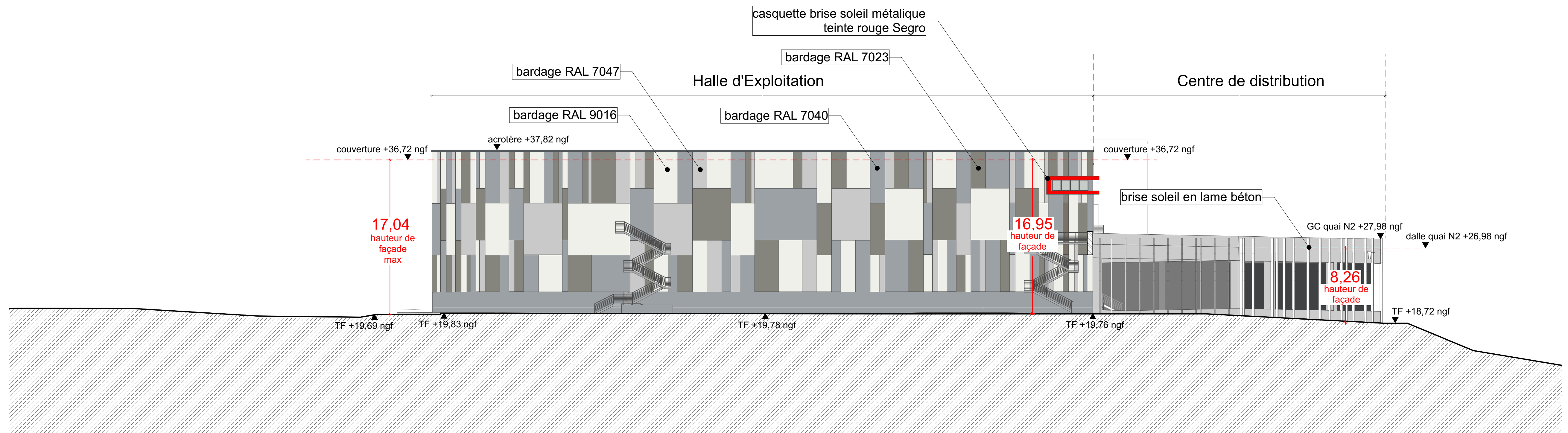
Facade Ouest - 1/250
