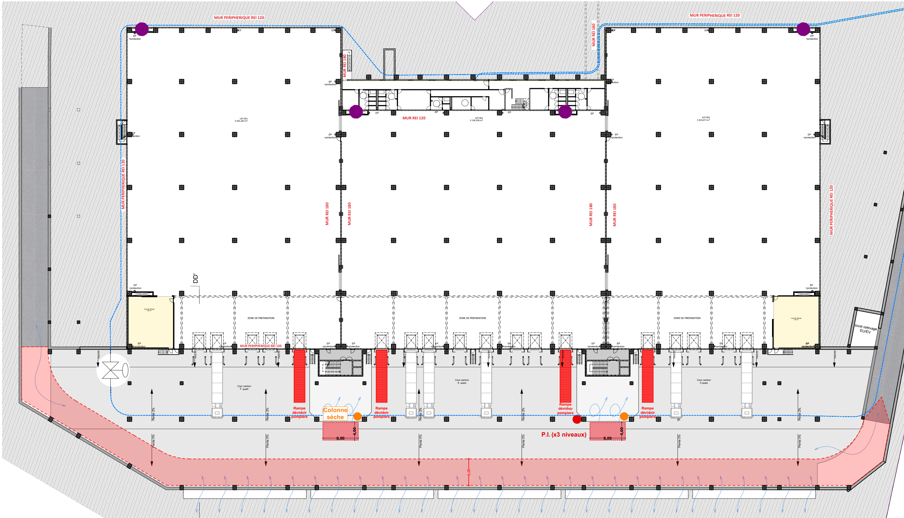
Extrait de plan N0 - Principe d'aération naturelle par cour anglaise, accès et patio
