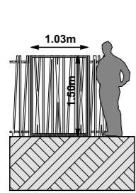
Portail remplissage à barreaudage type O'Bamboo à créer hauteur 1.50m teinte gris anthracite
