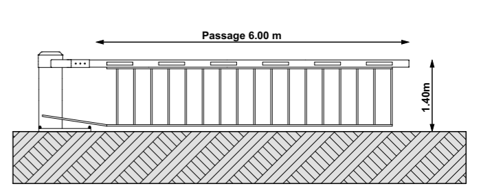
Barrière levante automatique à créer
