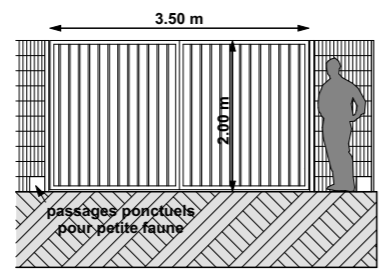
Portail à barreaudage à créer Hauteur 2m RAL 6005
