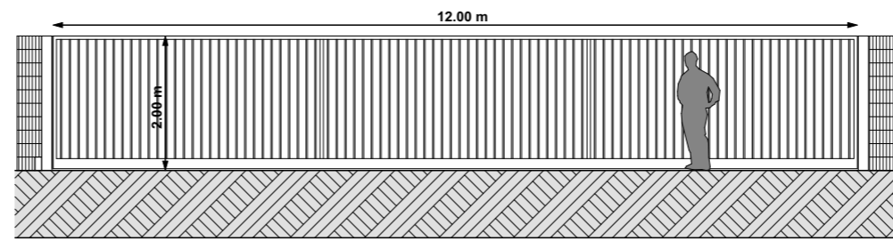
Portail à barreaudage coulissant à créer Hauteur 2m RAL 6005
