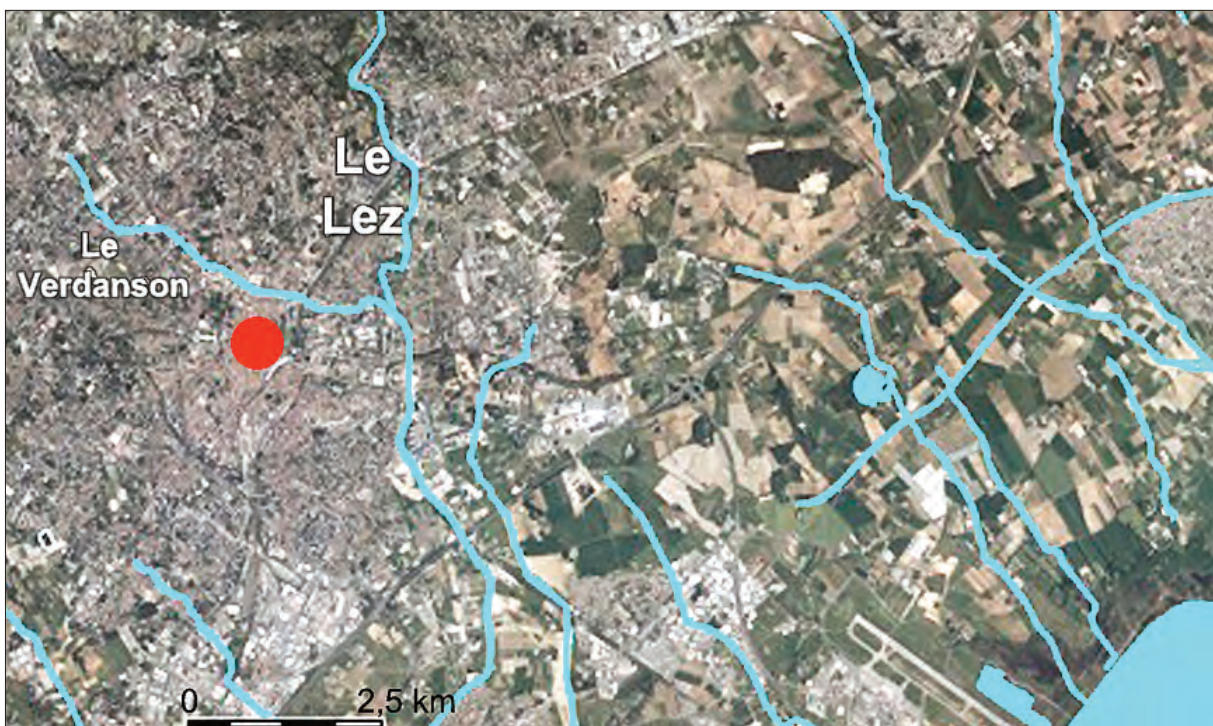
Réseau hydrographique.
