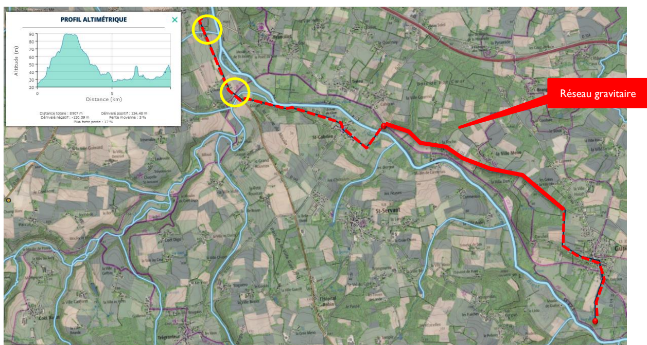
Figure 29 : proposition de tracé d'un réseau de transfert des eaux usées de Guillac sur la station de Josselin
