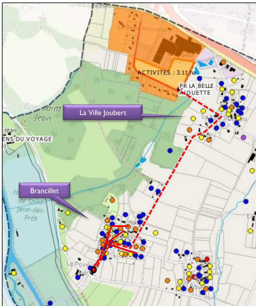
Figure 28 : proposition de raccordement des eaux usées de Brancillet au réseau collectif de Josselin
