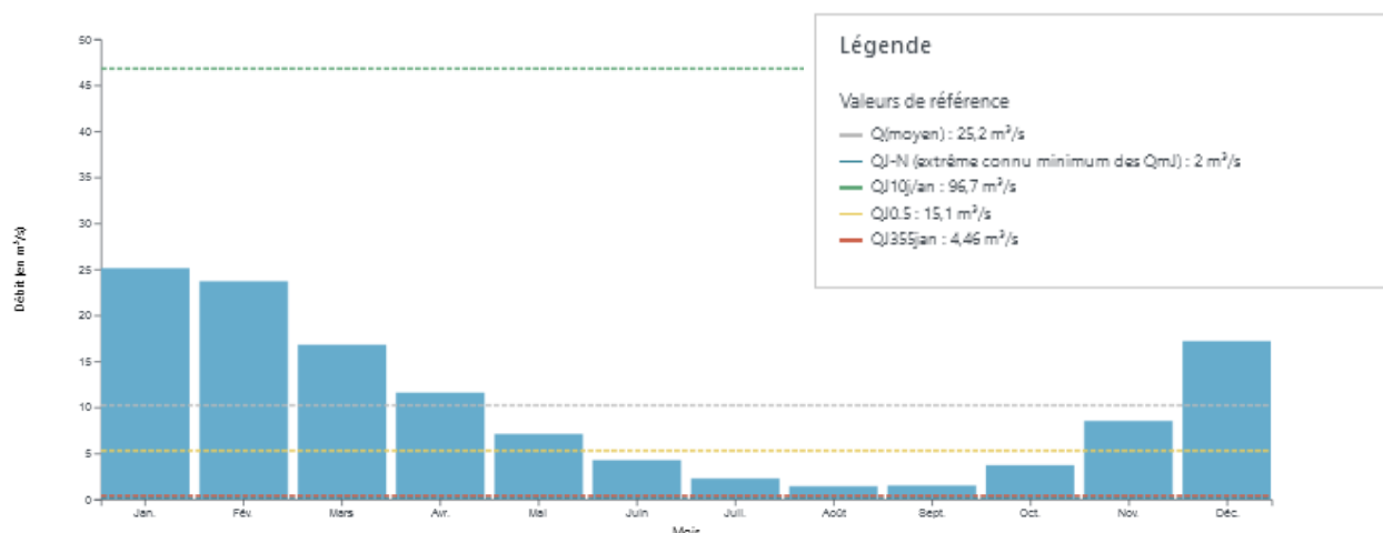
Figure 6 : Évolution moyenne des débits journaliers de l'Oust à Pleugriffet (907 km 2 ) (Banque hydro)
