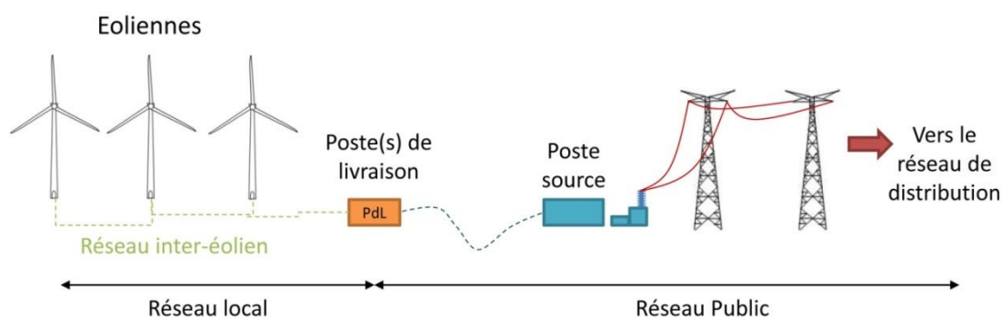
Figure 10 - Schéma de principe du raccordement électrique d'un parc éolien
