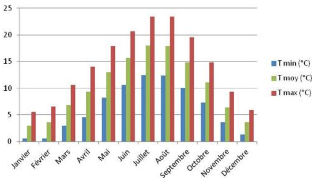
Figure 4 – Diagramme des températures mensuelles
