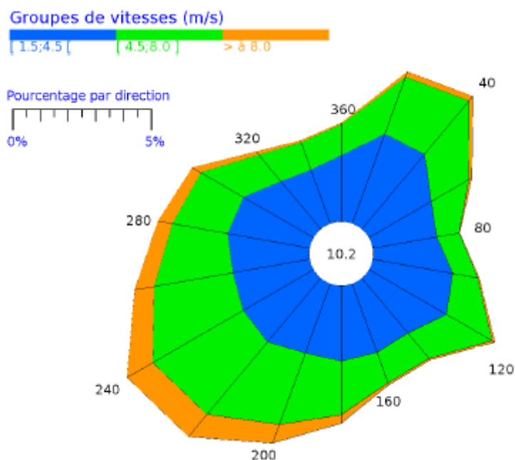
Figure 2 – Rose des vents à la station de Saint-Quentin
