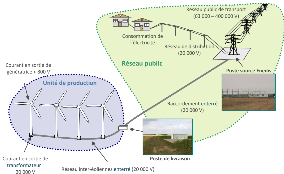
Figure 7 - Fonctionnement d'un parc éolien
