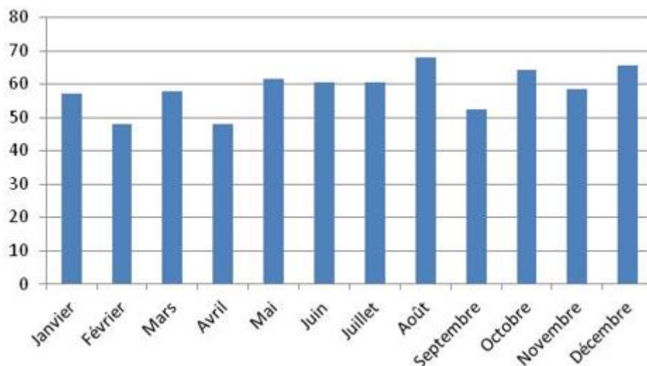
Figure 3 – Diagramme des précipitations à Saint-Quentin
