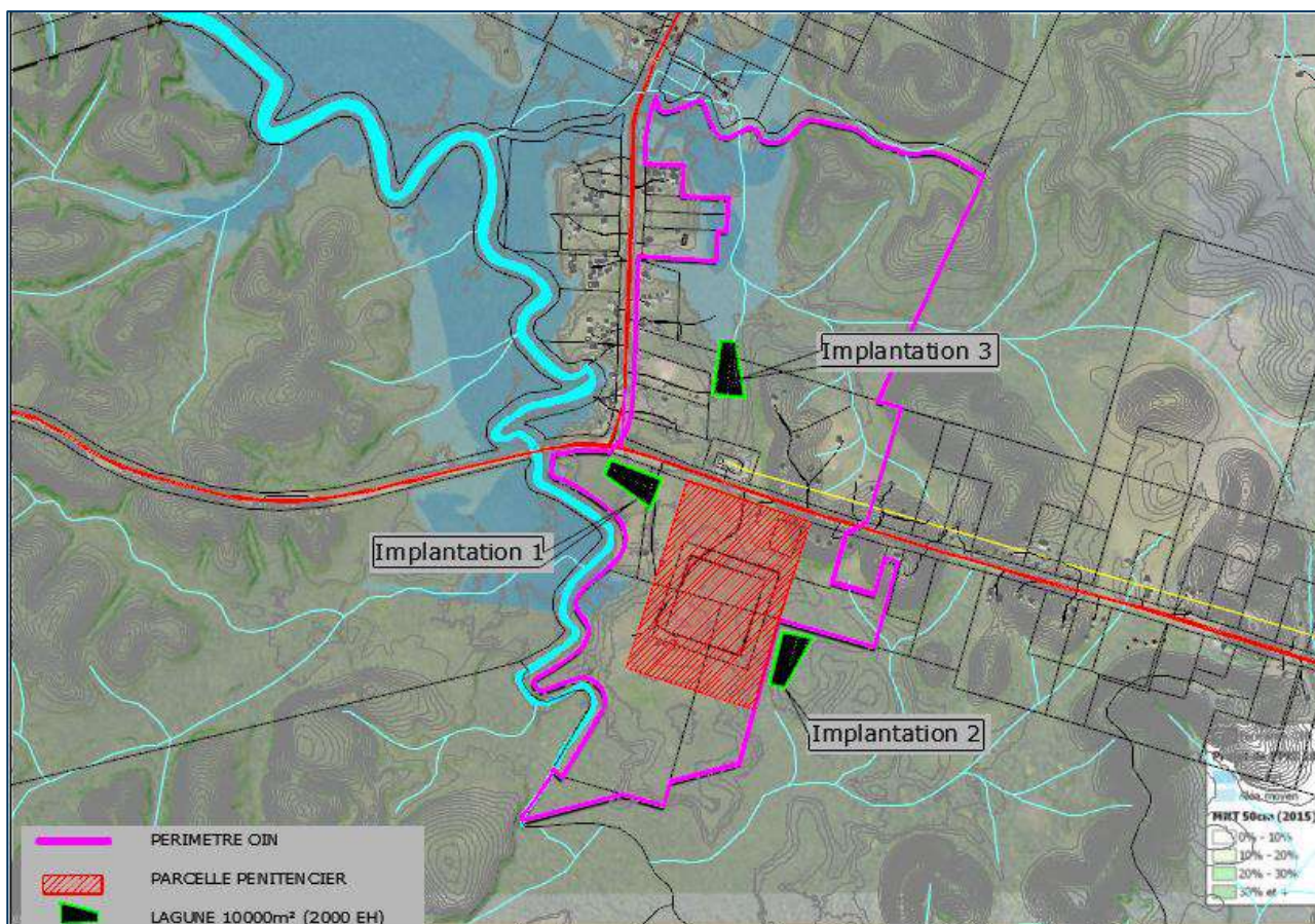
Figure 1 - Localisation des implantations possibles pour l'assainissement EU
