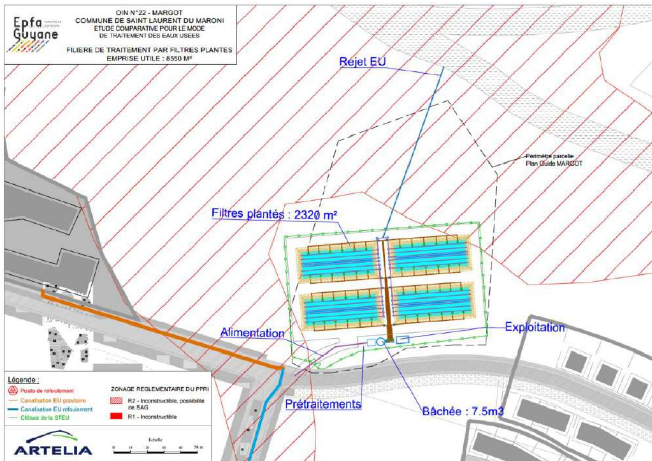
Figure 4 - Visuel Filtres Plantés Végétaux pour 2 900 EH
