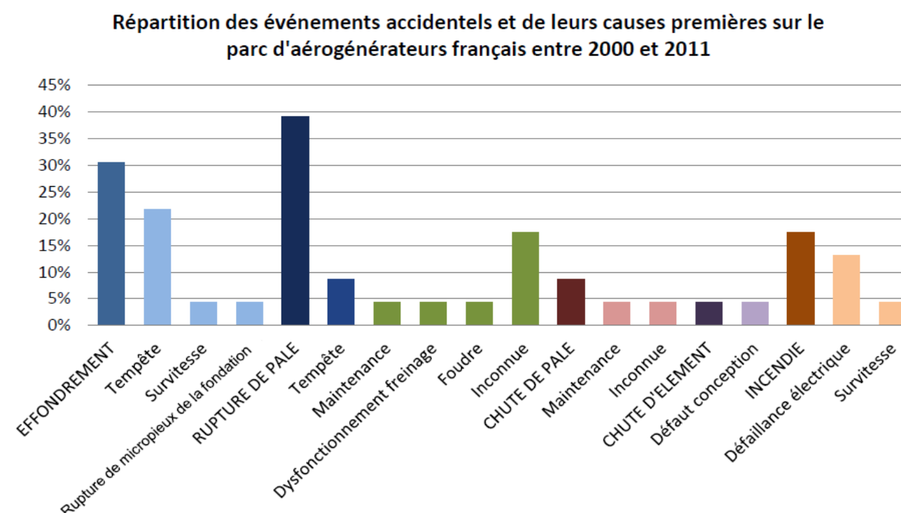
Figure 9 : Répartition des événements accidentels et de leurs causes premières sur le parc éolien français entre 2000 et 2011 (source : SER/FEE/INERIS, 2011)
