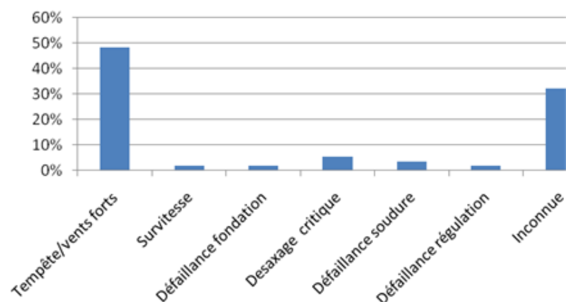
Figure 10 : Répartition des événements accidentels dans le monde entre 2000 et 2011 (source : SER/FEE/INERIS, 2012)
