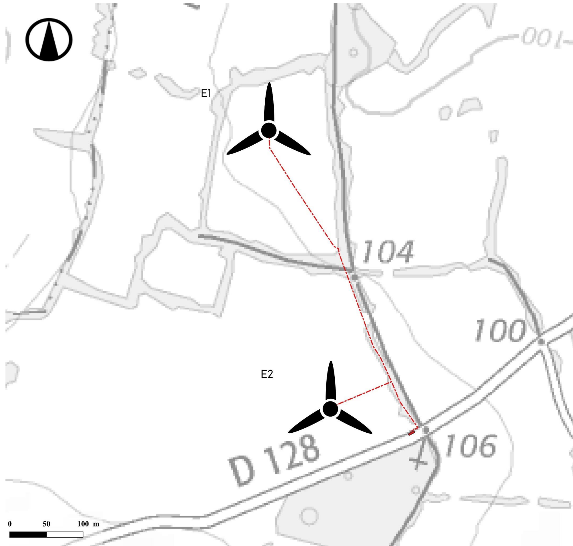
Carte 11 : Raccordement inter-éolien
