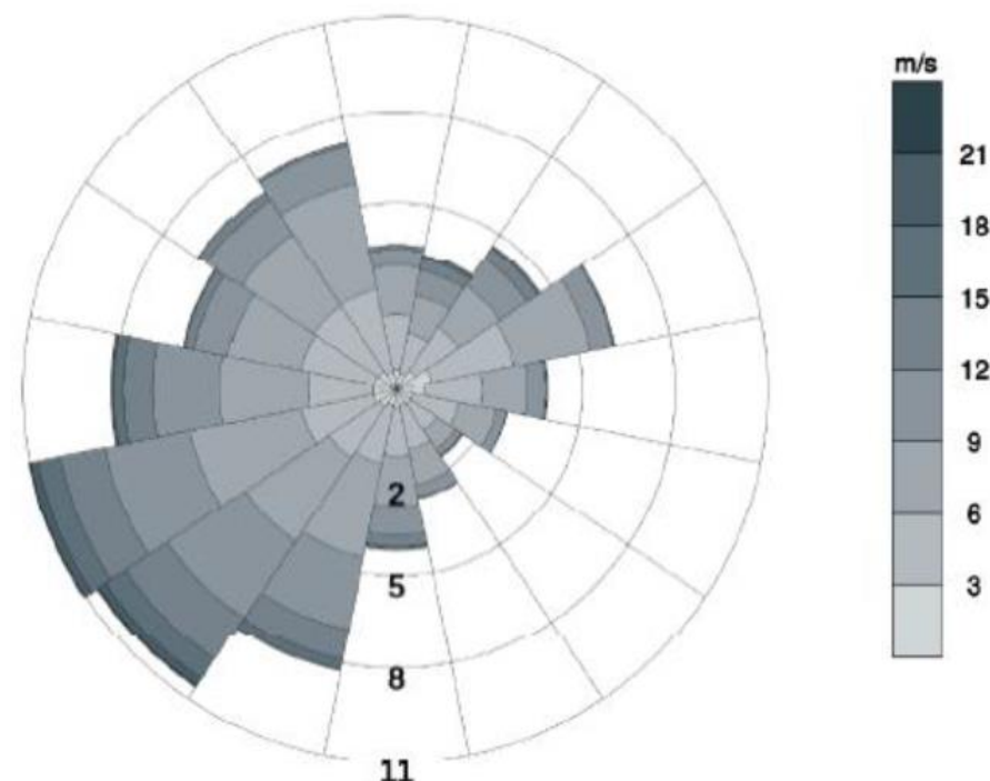
Figure 4 : Rose des vents sur le site éolien de La Grande Lande (source : ORFEA Acoustique, 2021)
