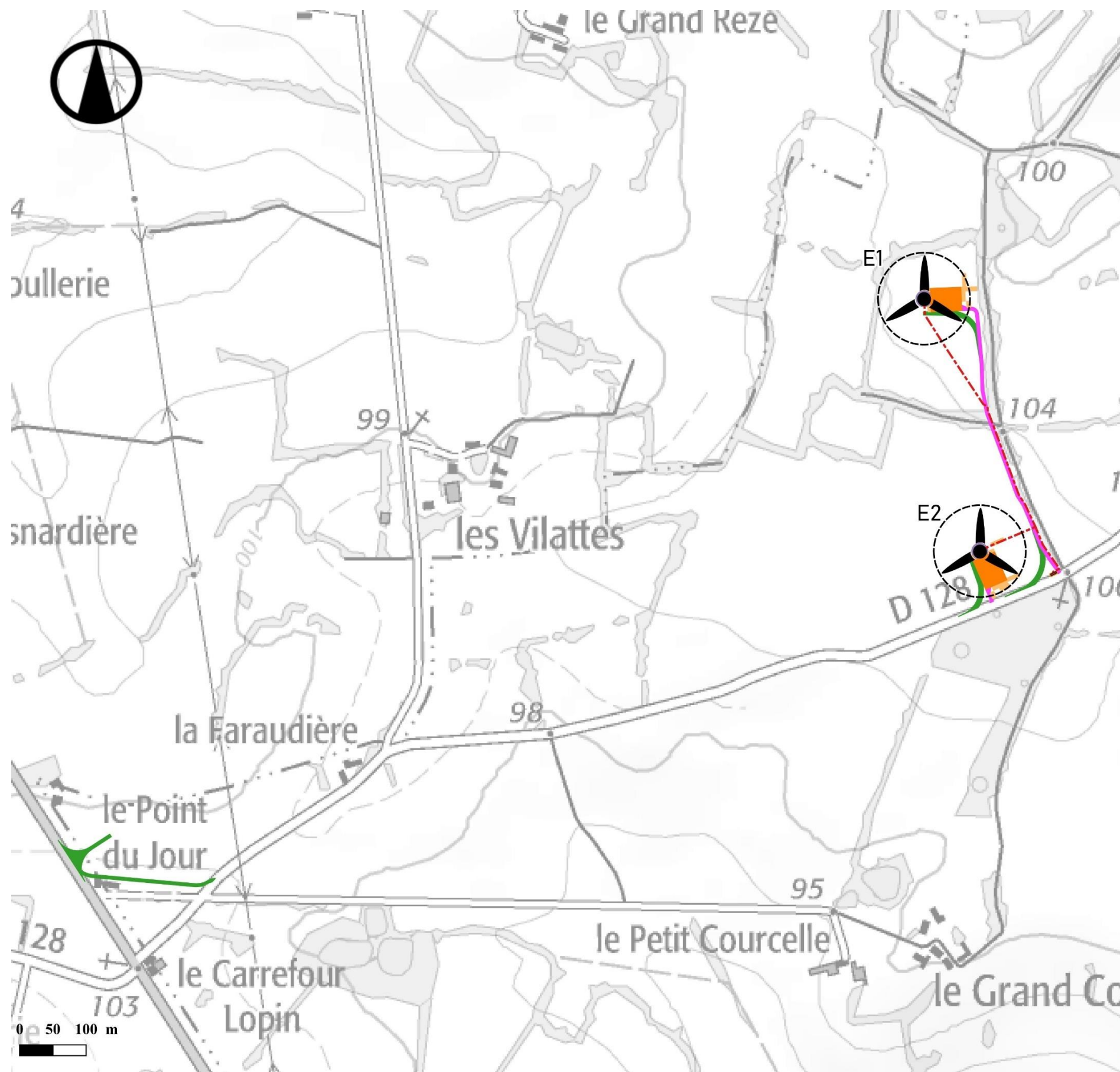
Carte 10 : Plan de l'installation et des aménagements
