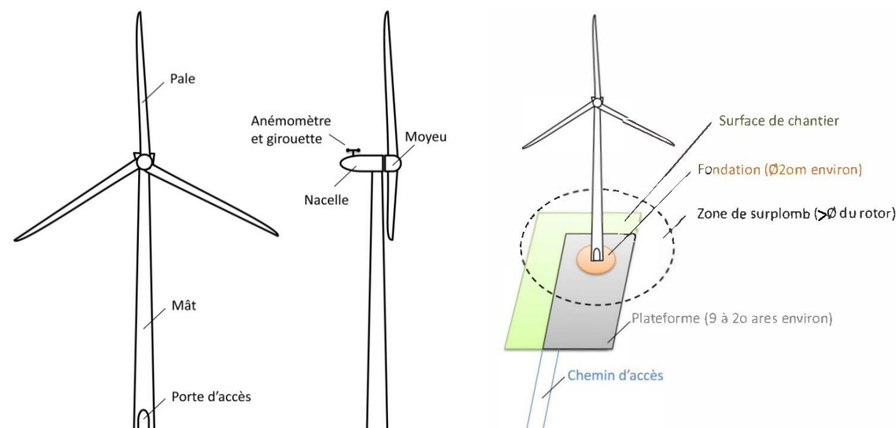
Figure 5 : Schéma simplifié d'un aérogénérateur (à gauche) - Illustration des emprises au sol d'une éolienne (à droite) (Les dimensions sont données à titre d'illustration pour une éolienne d'environ 150 m de hauteur totale) (source : Guide de l'INERIS, mai 2012)
