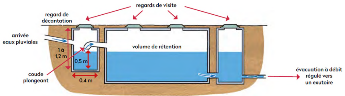
Figure 18 : Schéma de principe d'un bassin enterré
