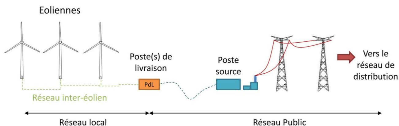
Figure 12 : Schéma de raccordement électrique d'un parc éolien
