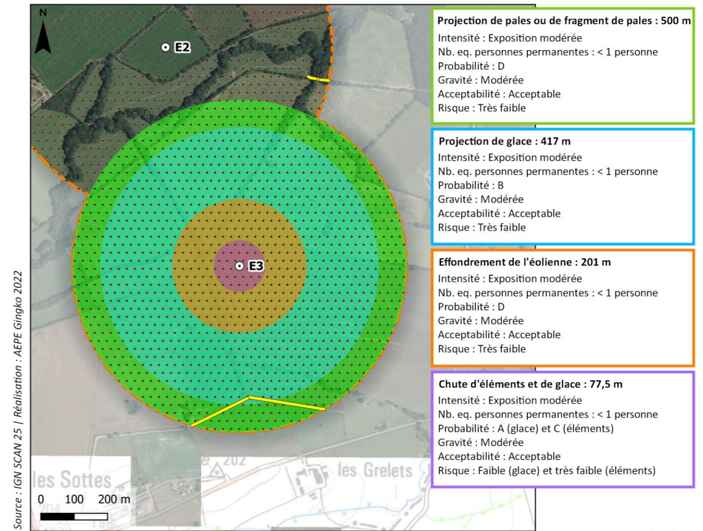
Zones d'effets des risques étudiés pour l'éolienne E3
