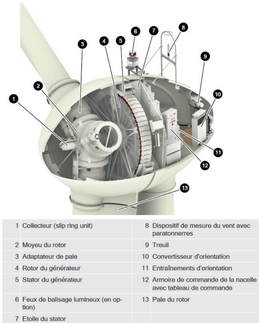
Figure 7 : Dessin schématique d'une nacelle (Source : ENERCON)
