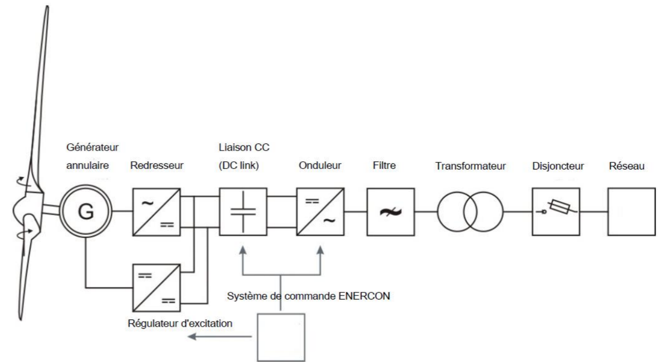
Figure 8 : Schéma électrique simplifié d'une éolienne ENERCON (Source : ENERCON)
