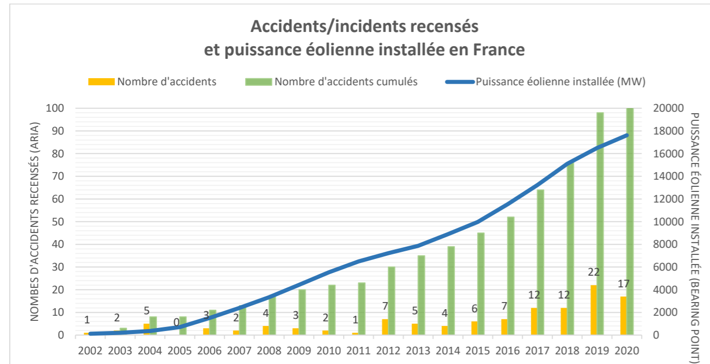
Figure 16 : Le nombre d'accidents éoliens recensés par la base ARIA entre 2002 et 2020 en France (Source : ARIA)
