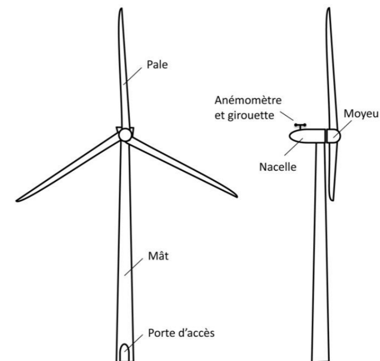
Figure 4 : Schéma simplifié d'un aérogénérateur (Source : Nordex)
