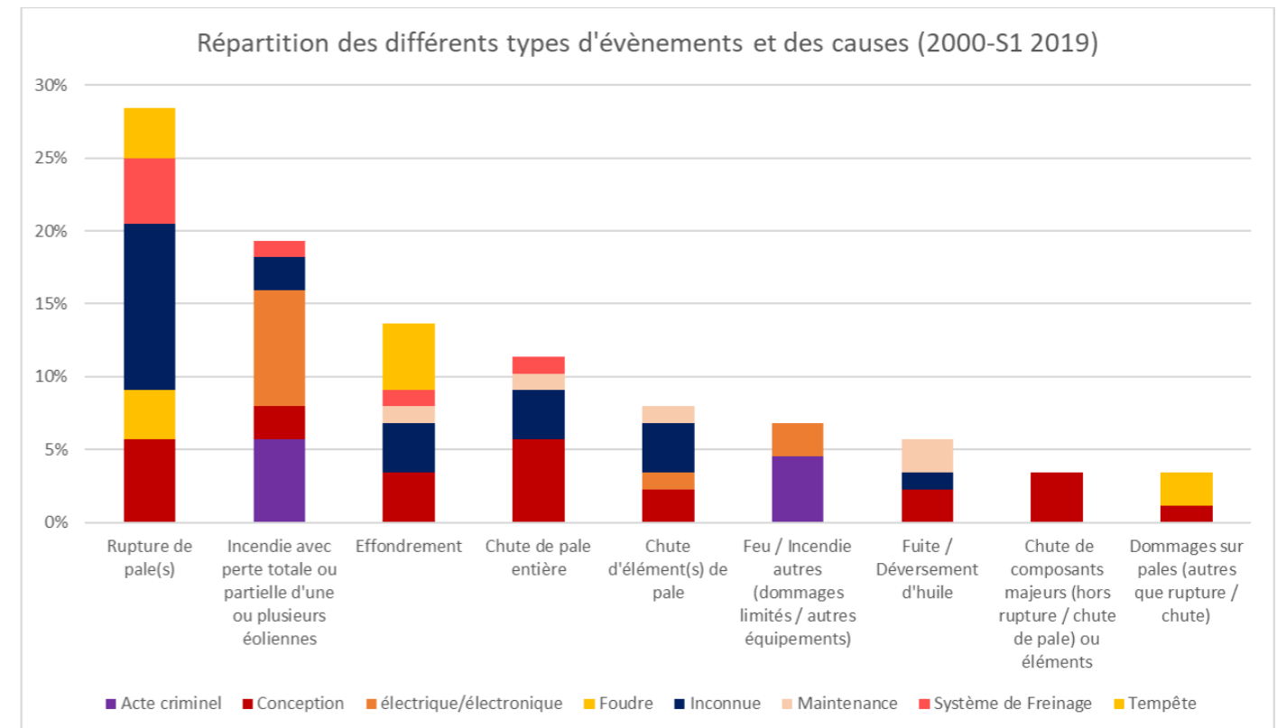
Figure 13 : Les causes premières des accidents d'aérogénérateurs en France (Source : FEE)
