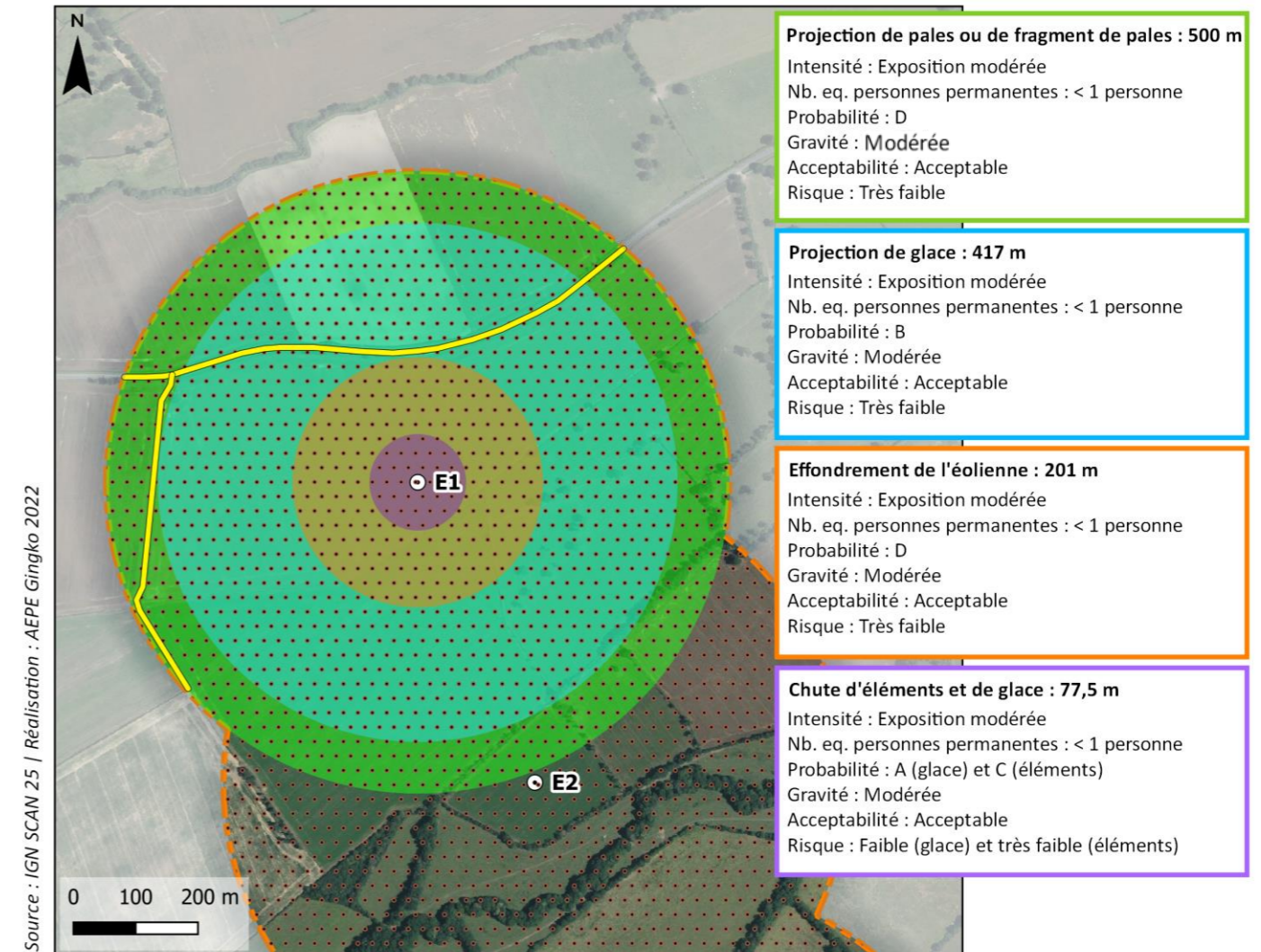
Zones d'effets des risques étudiés pour l'éolienne E1
