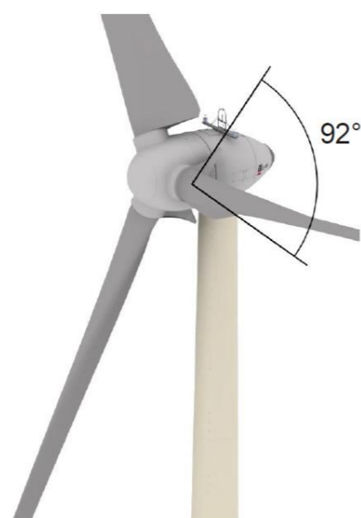
Figure 10 : Mise en drapeau des pales lors de l'arrêt automatique ou manuel de l'éolienne (Source : ENERCON)
