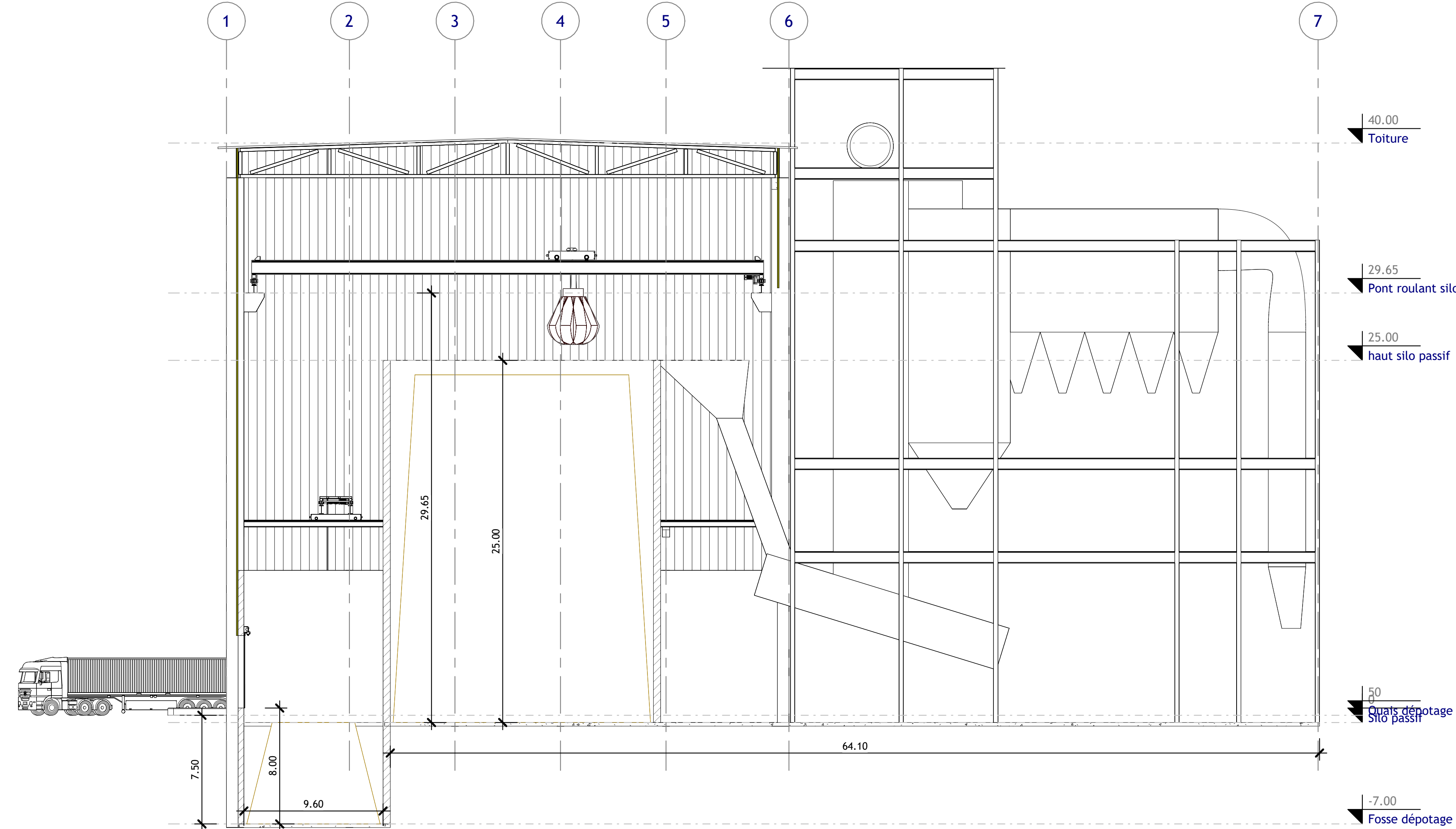
Coupe B-B
