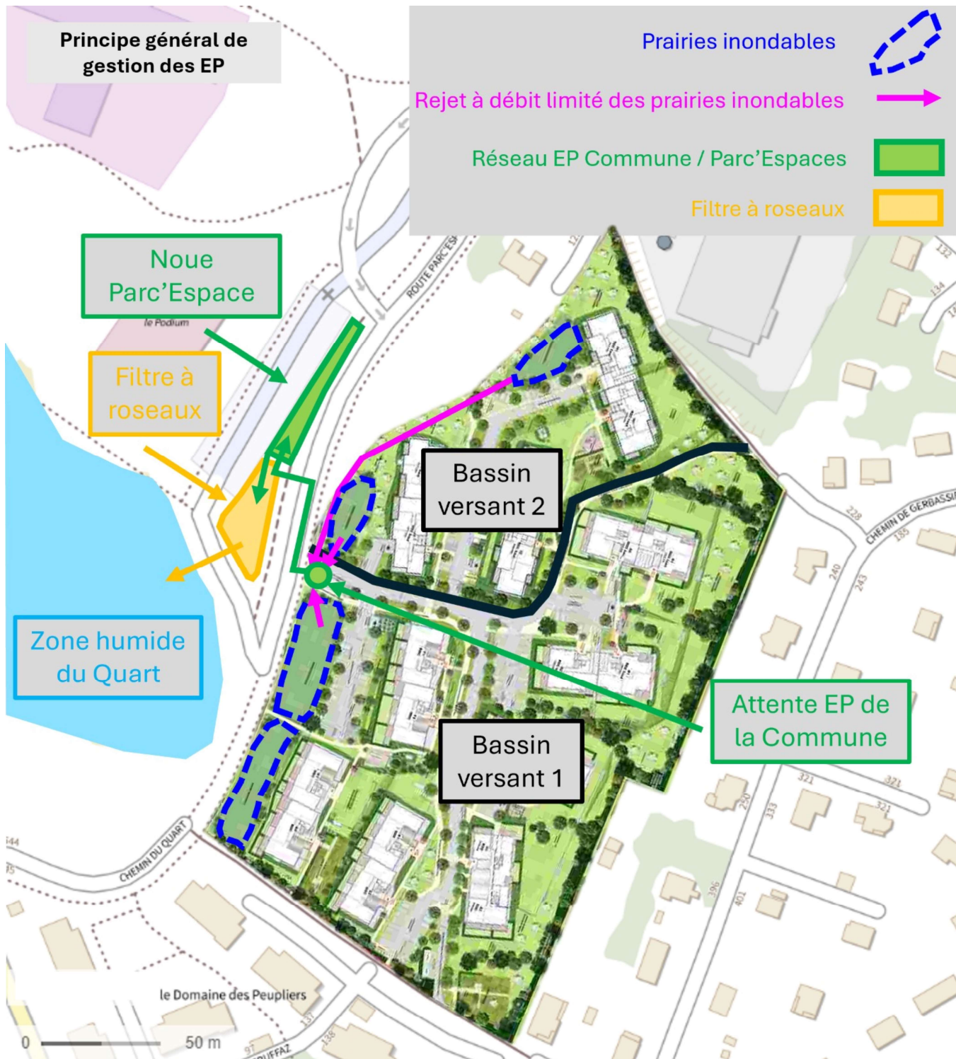
Principe général de gestion des eaux pluviales
