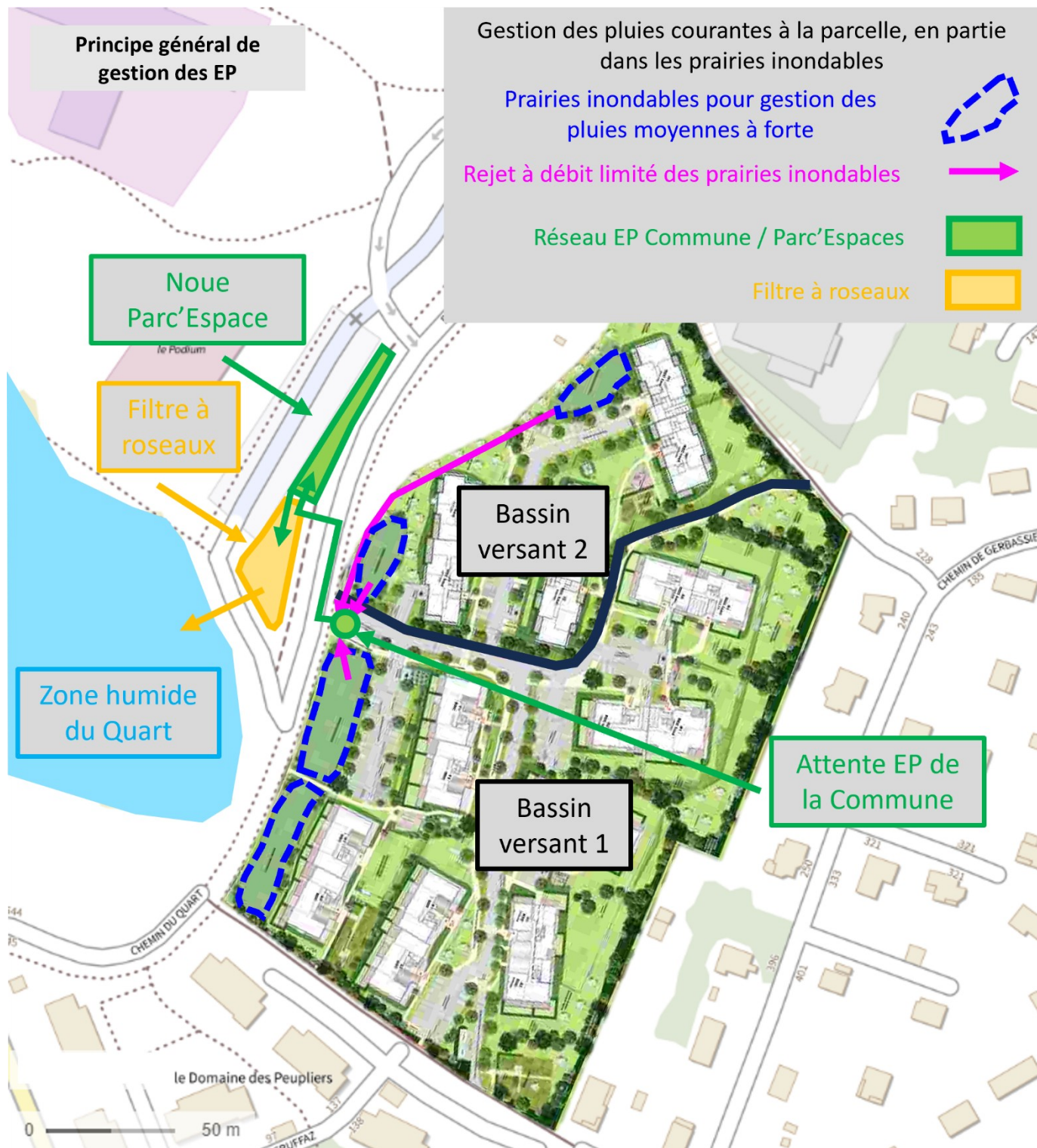
Schéma exutoire EP
