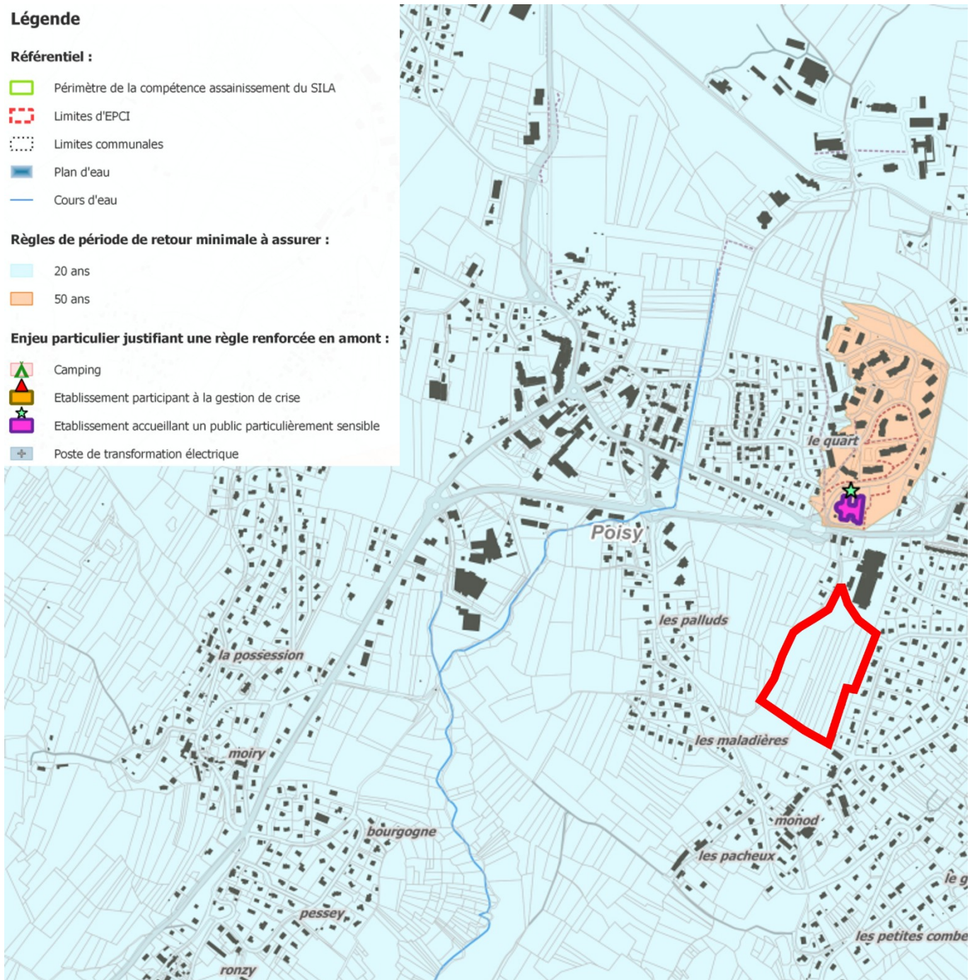
Extrait de la carte de période de retour d'insuffisance à assurer
