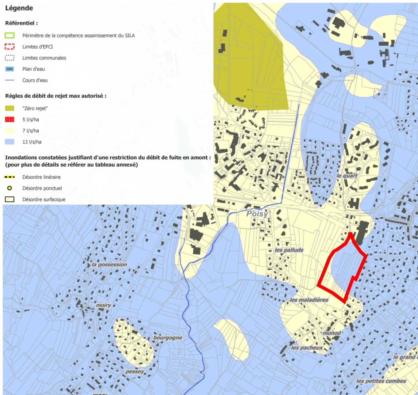
Extrait de la carte des débits de rejets maximum autorisés
