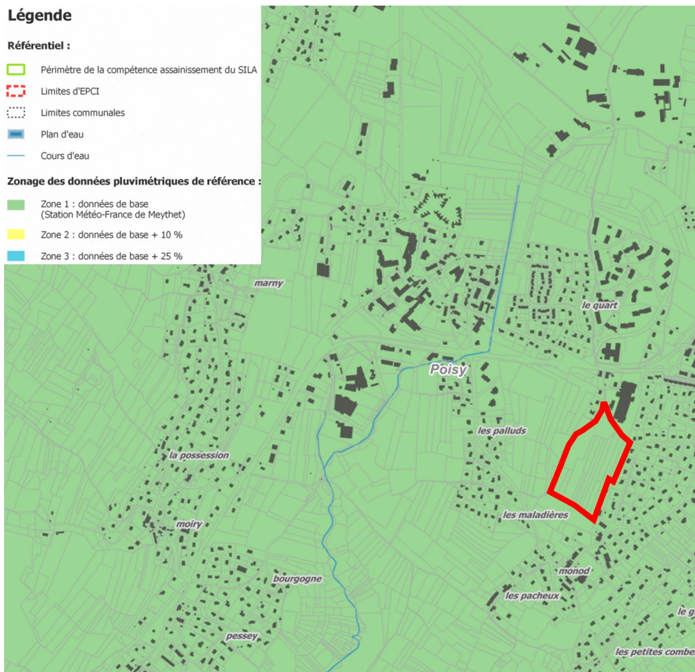
Extrait de la carte des coefficients pluviométriques
