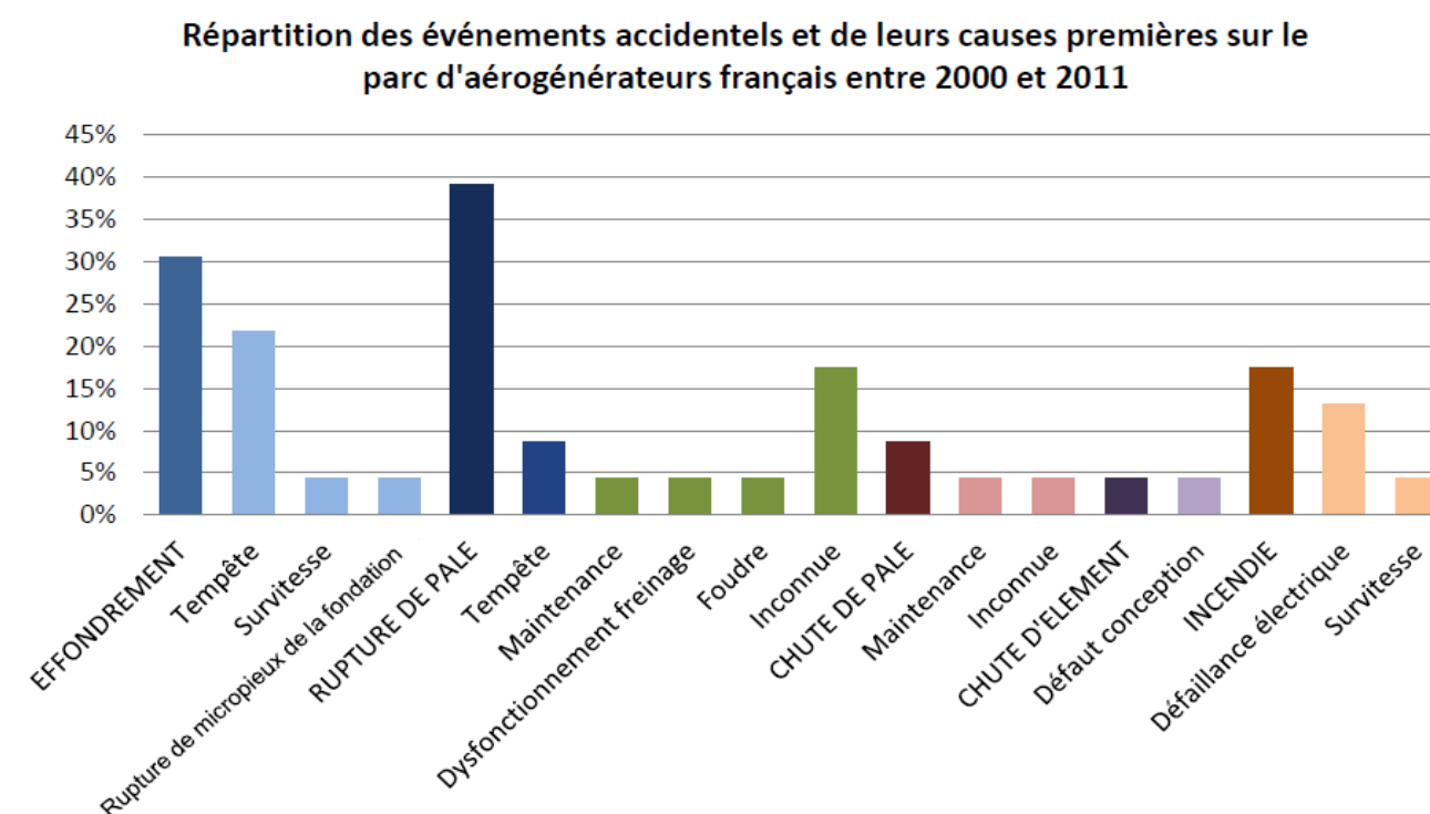
Figure 8 : Répartition des événements accidentels et de leurs causes premières sur le parc éolien français entre 2000 et 2011 (source : SER/FEE/INERIS, 2011)
