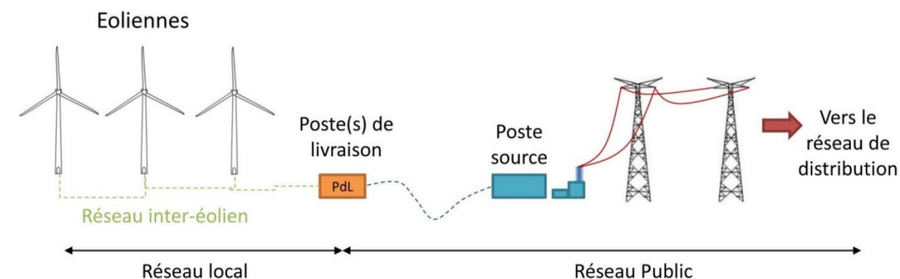
Figure 6 : Raccordement électrique des installations (source : INERIS/SER/FEE, 2012)
