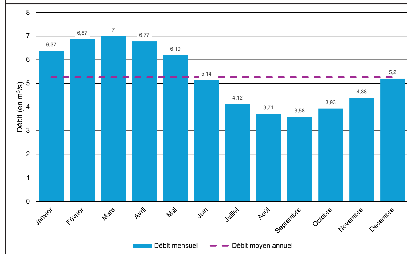
Figure 28 : Débit mensuel de la Vanne à Pont-sur-Vanne de 1961 à 2024
