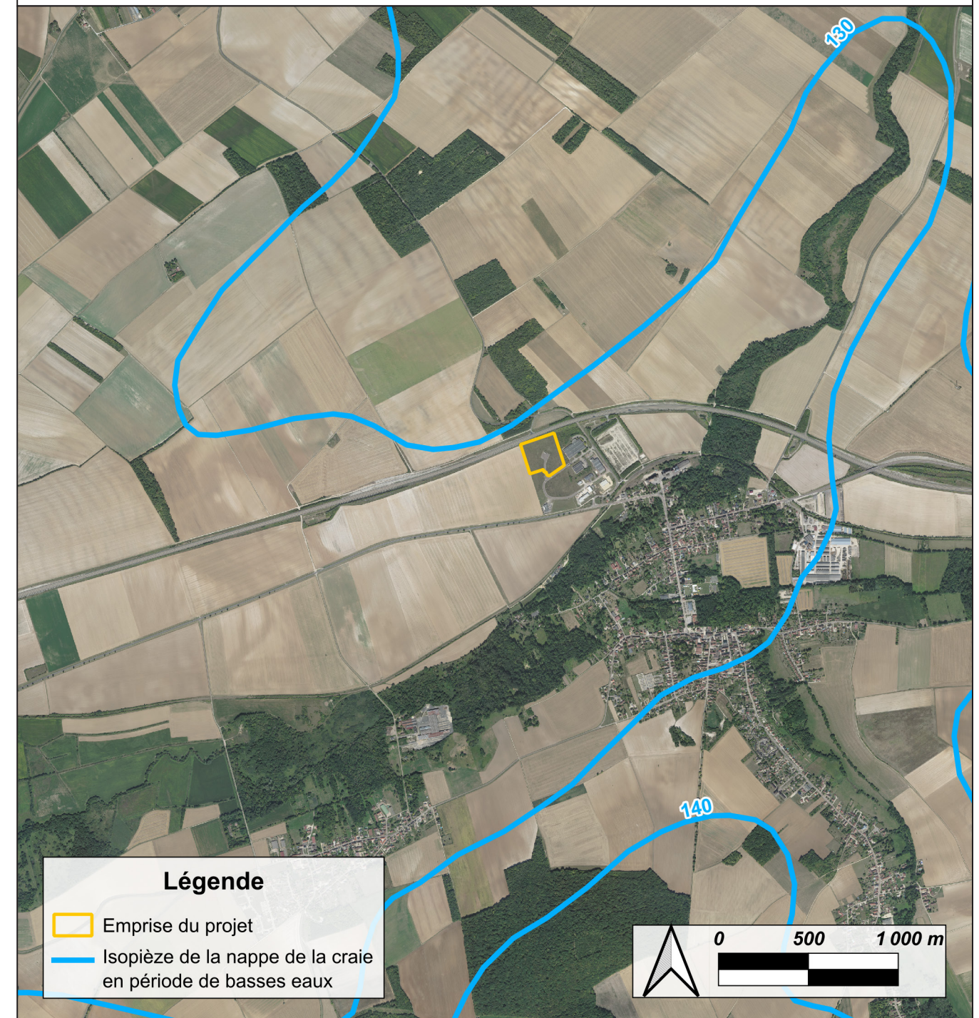
Figure 24 : Isopièzes de la nappe de la craie en période de basses eaux
