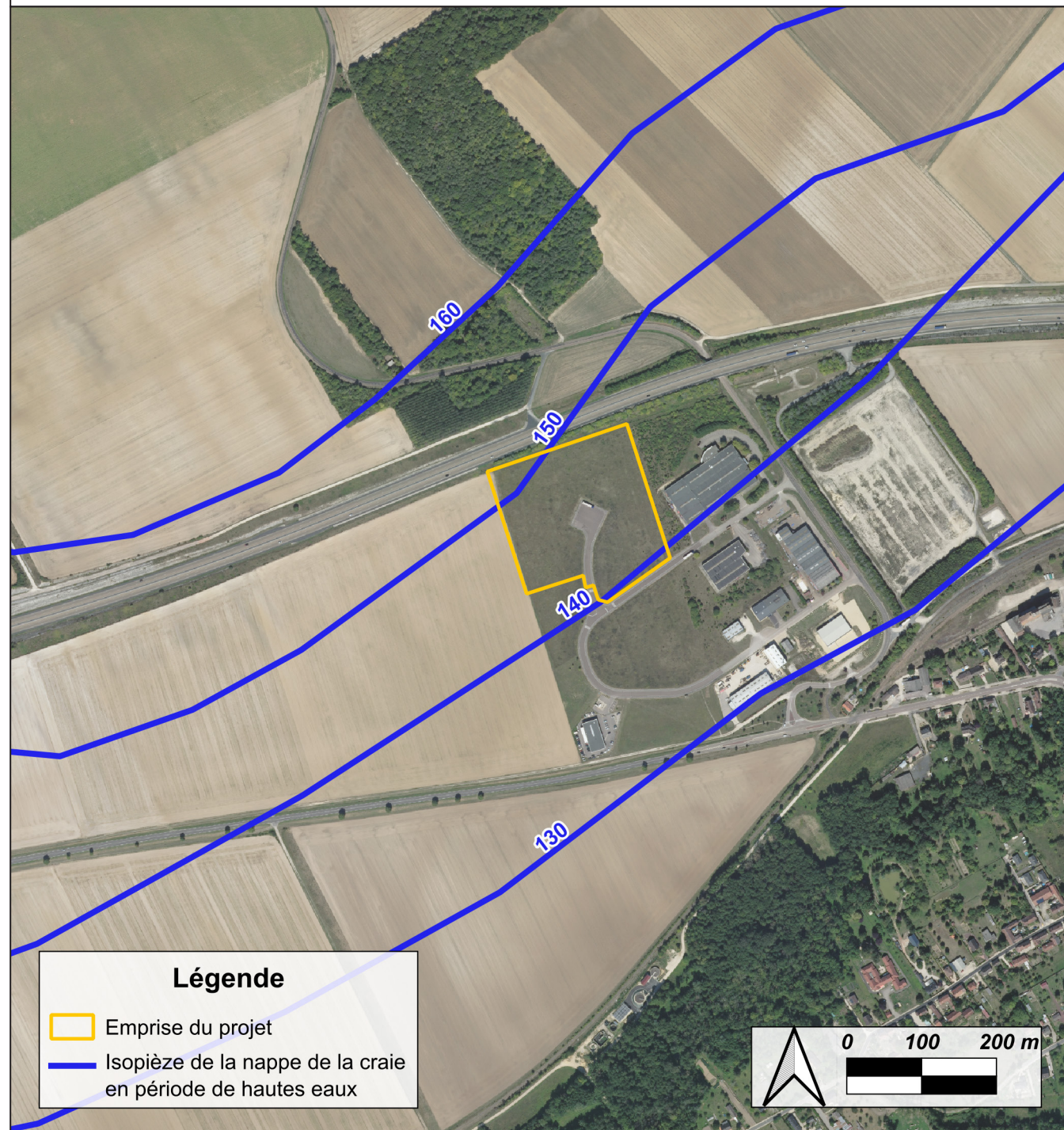
Figure 23 : Isopièzes de la nappe de la craie en période de hautes eaux
