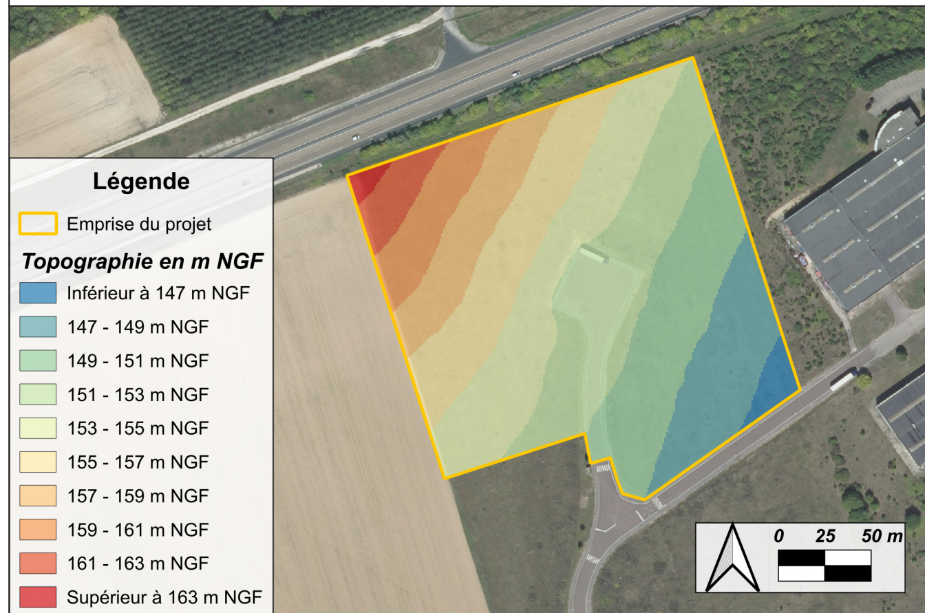
Figure 22 : Topographie au niveau du site du projet
